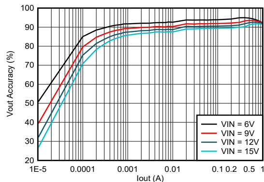
效率与输出电流间的关系 (频率为 1.0MHz, V OUT = 3.3V, 自动 PFM/PWM)
