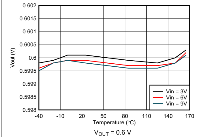
图 7-9. Output Voltage Accuracy - VSET Selected
