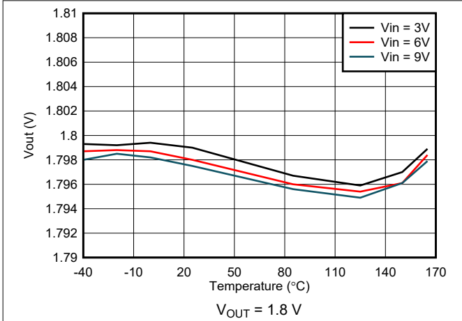
图 7-7. Output Voltage Accuracy - VSET Selected
