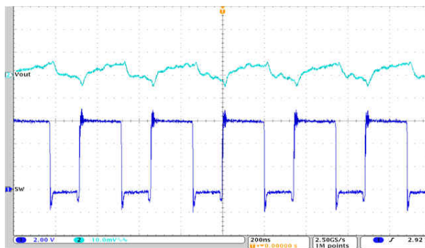
图 9-76. Output Voltage Ripple
