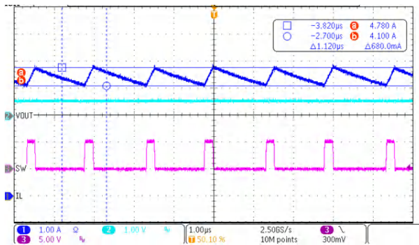
图 9-78. Output Voltage Ripple
