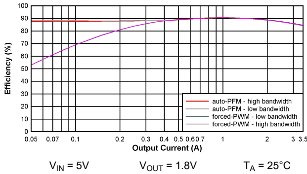
图 6-1. BUCK1 效率
