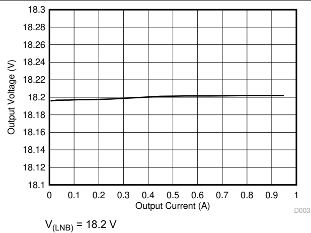
图 6-3. Load Regulation
