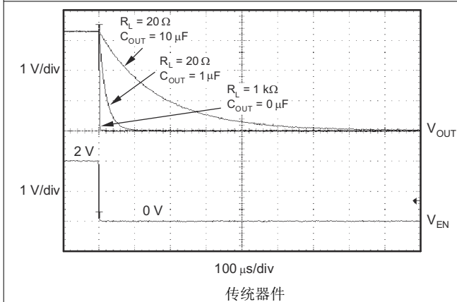
图 5-41. TPS73133 关断响应
