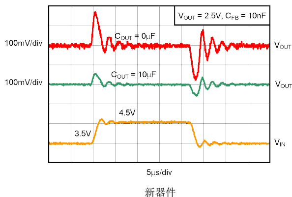
图 5-54. TPS73101 线路瞬态, 可调节版本
