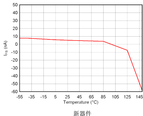
图 5-50. TPS73101 I_{FB} 与温度间的关系
