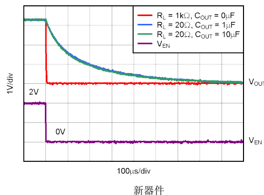
图 7-6. TPS73133 关断响应
