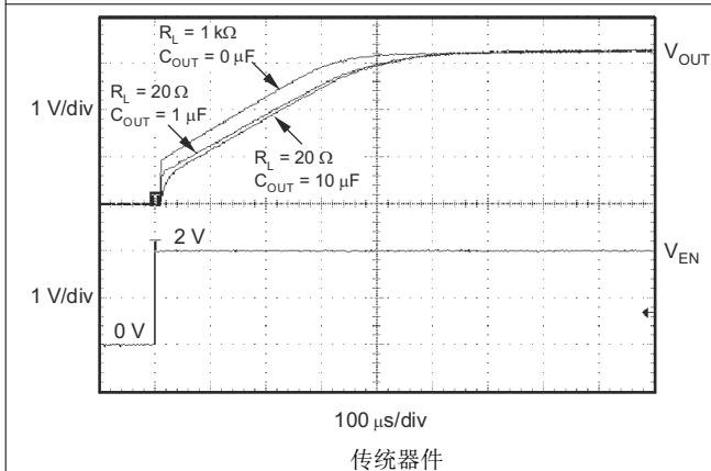
图 5-39. TPS73133 导通响应
