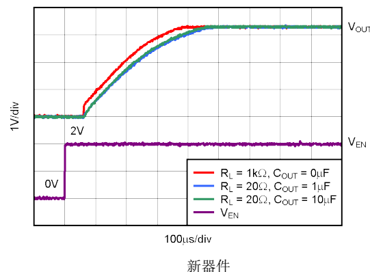
图 7-4. TPS73133 导通响应
