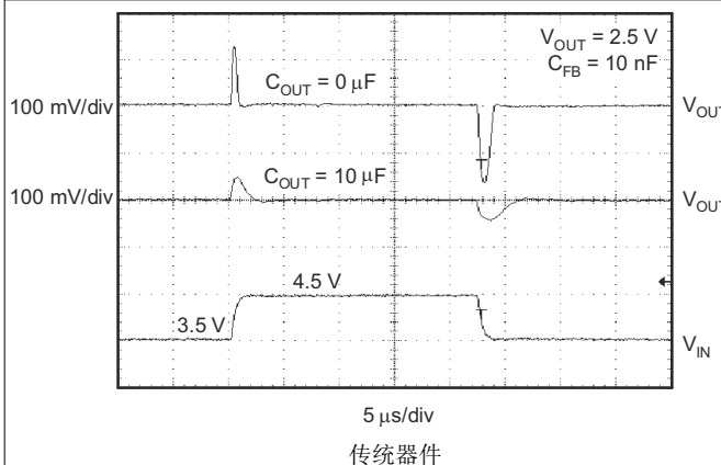
图 5-53. TPS73101 线路瞬态, 可调节版本
