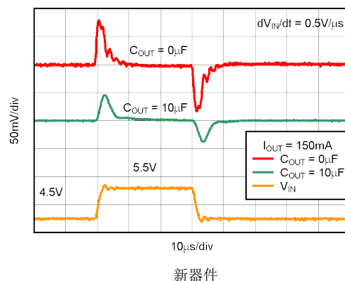
图 5-38. TPS73133 线路瞬态响应
