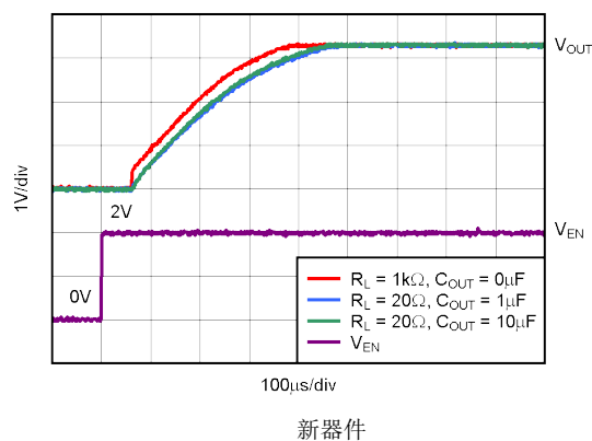
图 5-40. TPS73133 导通响应
