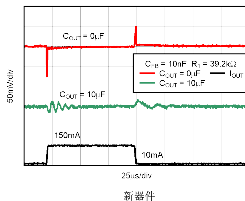
图 5-52. TPS73101 负载瞬态, 可调节版本
