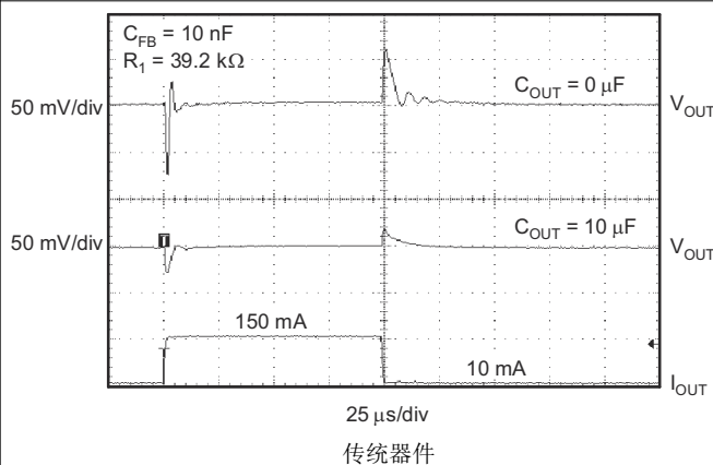
图 5-51. TPS73101 负载瞬态, 可调节版本
