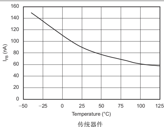
图 5-49. TPS73101 I_{FB} 与温度间的关系
