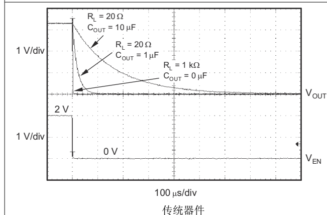
图 7-5. TPS73133 关断响应
