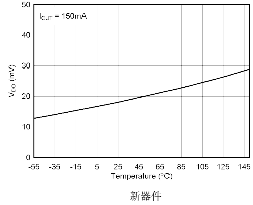
图 5-8. 压降电压与温度间的关系
