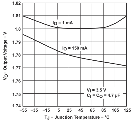
图 5-9. TPS76318-Q1 输出电压与自然通风温度间的关系 (旧芯片)
