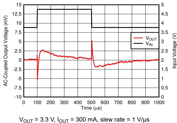
图 6-17. Line Transient
