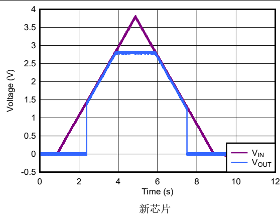
图 5-28. 上电和断电
