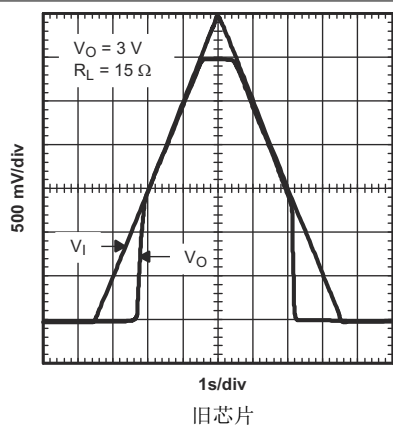
图 5-27. 上电和断电
