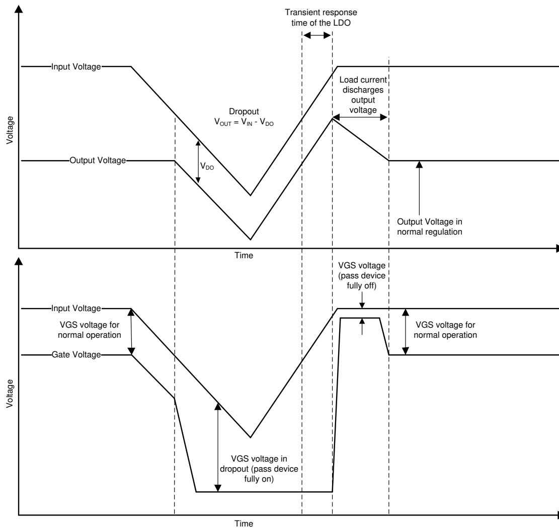
图 7-2. 压降产生的线路瞬变
