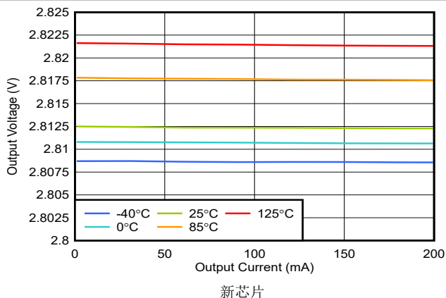
图 5-2. TPS793-Q1 输出电压与输出电流间的关系
