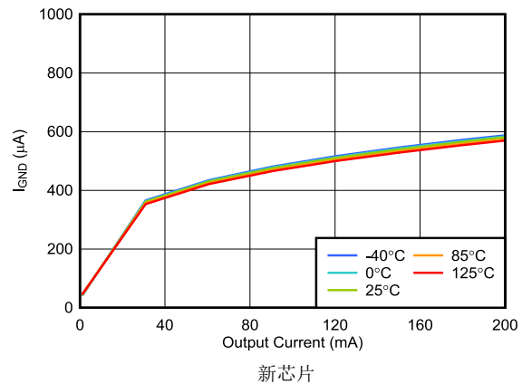
图 5-6. TPS793-Q1 接地电流与结温间的关系
