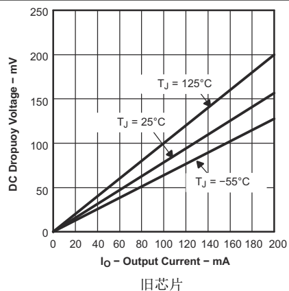
图 5-29. 压降电压与输出电流间的关系
