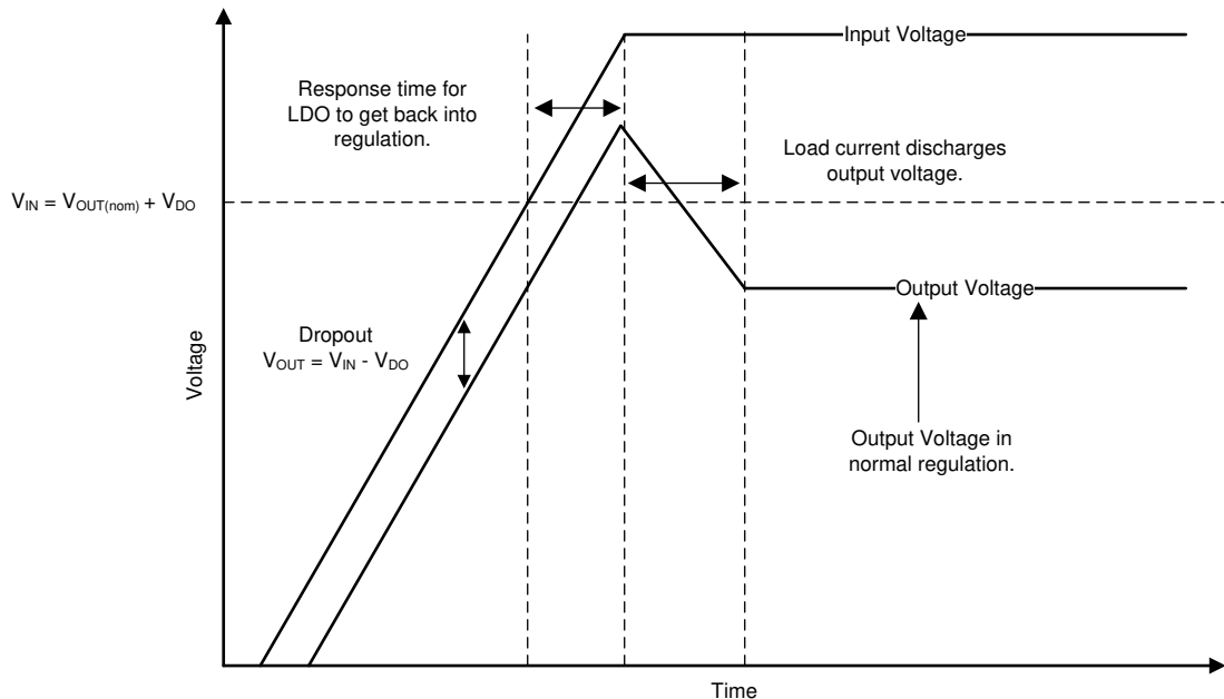
图 7-1. 启动至压降
