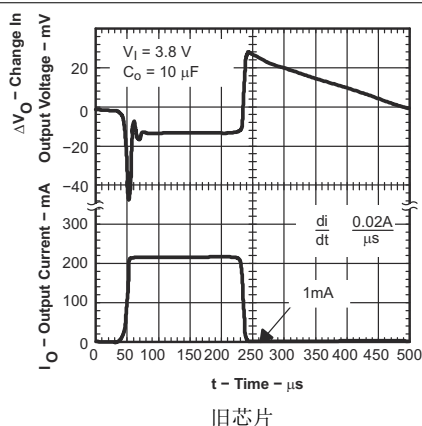
图 5-25. TPS793-Q1 负载瞬态响应
