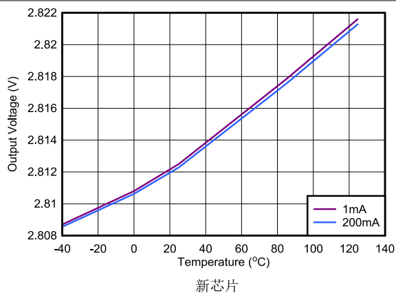
图 5-4. TPS793-Q1 输出电压与结温间的关系
