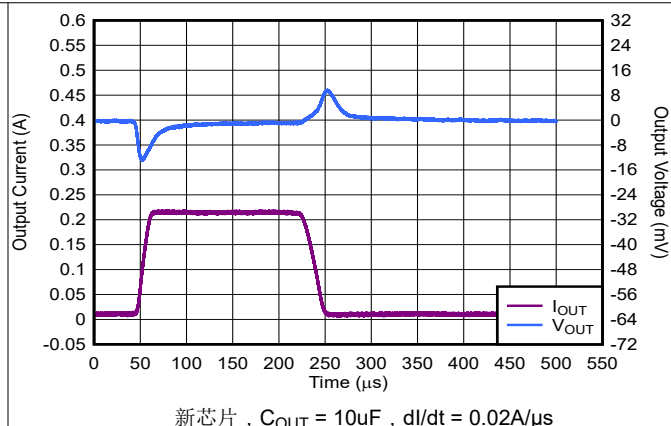
图 5-26. TPS79328 负载瞬态响应
