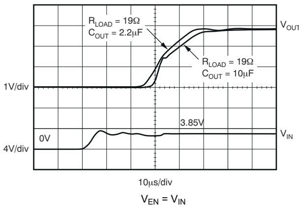
图 6-23. TPS799285 Turn-On Response
