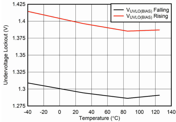
图 6-13. V_{BIAS} UVLO vs Temperature
