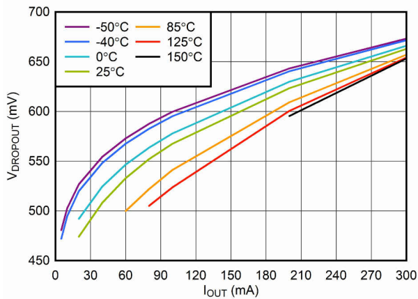
图 6-5. V_{BIAS} Dropout Voltage vs I_{OUT}
