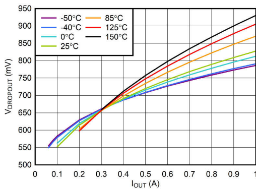
图 6-5. V_{BIAS} Dropout Voltage vs I_{OUT}
