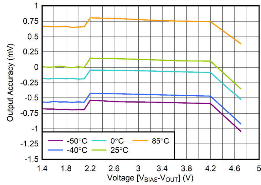
图 6-2. Output Voltage Accuracy vs V_{BIAS}
