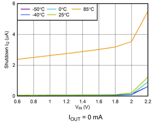
图 6-8. V_{\text{IN}} Shutdown I_{\text{Q}} vs V_{\text{IN}}
