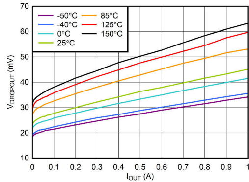
图 6-4. V_{IN} Dropout Voltage vs I_{OUT}
