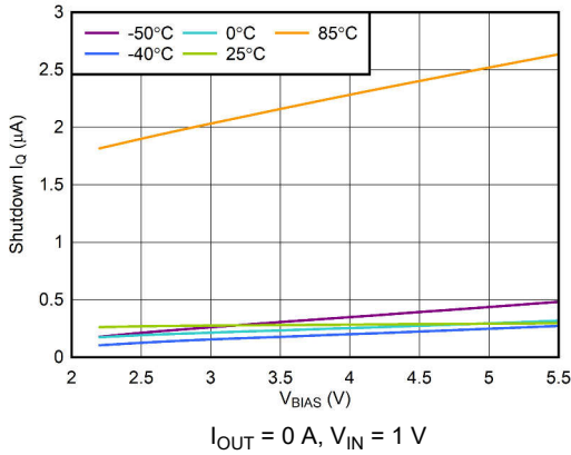
图 6-9. V_{\text{BIAS}} Shutdown I_{\text{Q}} vs V_{\text{BIAS}}
