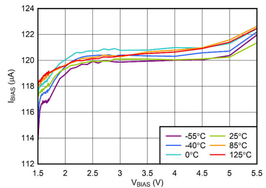
图 6-6. V_{BIAS} Input Current vs V_{BIAS}
