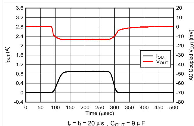
图 5-23. 从 100µA 至 1A 的负载瞬态
