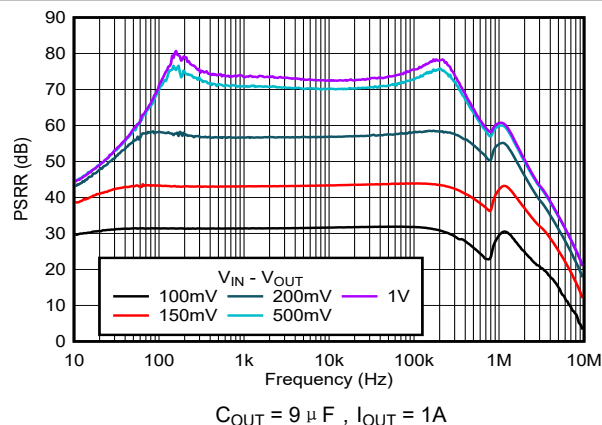
图 5-26. PSRR 与频率和 V_{\text{IN}} - V_{\text{OUT}} 间的关系
