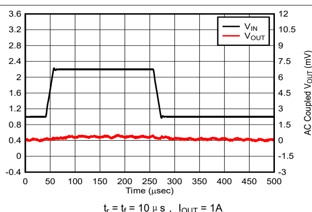
图 5-20. 从 1V 至 2.2V 的线路瞬态
