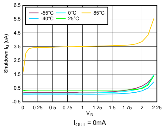
图 5-8. V_{\text{IN}} 关断 I_Q 与 V_{\text{IN}} 间的关系
