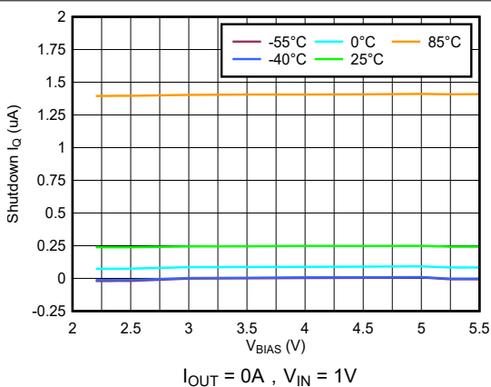
图 5-9. V_{\text{BIAS}} 关断 I_Q 与 V_{\text{BIAS}} 间的关系
