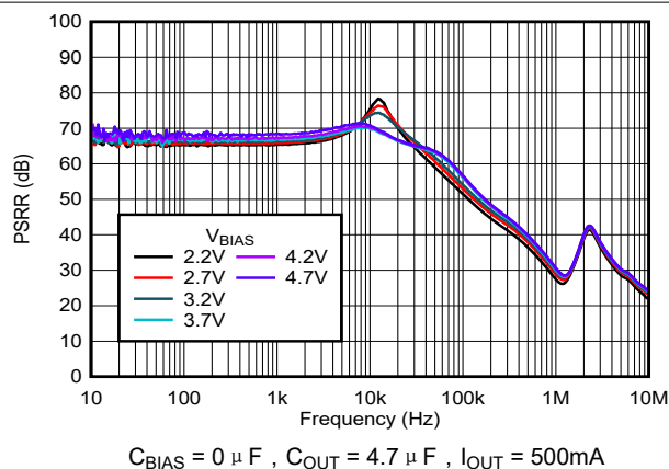
图 5-29. PSRR 与频率和 V_{\text{BIAS}} - V_{\text{OUT}} 间的关系
