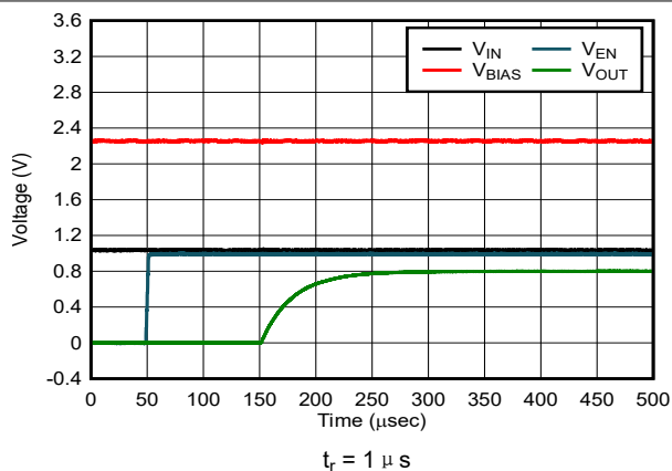
图 5-16. 在先施加 V_{\text{IN}} 和 V_{\text{BIAS}} 后施加 V_{\text{EN}} 的情况下启动
