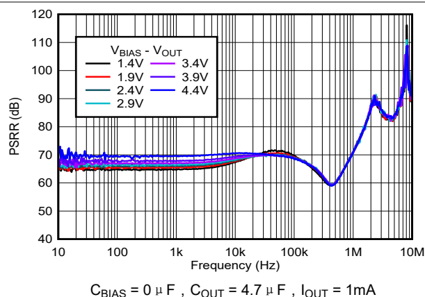
图 5-28. PSRR 与频率和 V_{\text{BIAS}} - V_{\text{OUT}} 间的关系
