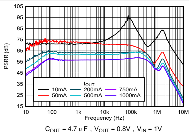
图 5-27. PSRR 与频率和 I_{\text{OUT}} 间的关系
