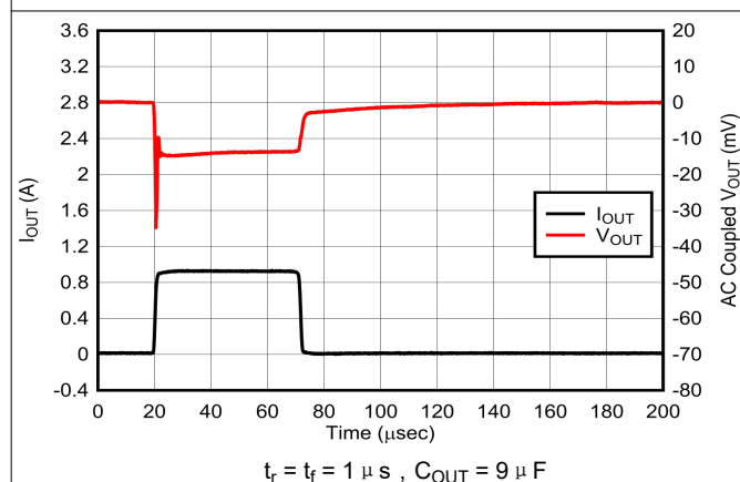
图 5-21. 从 100µA 至 1A 的负载瞬态
