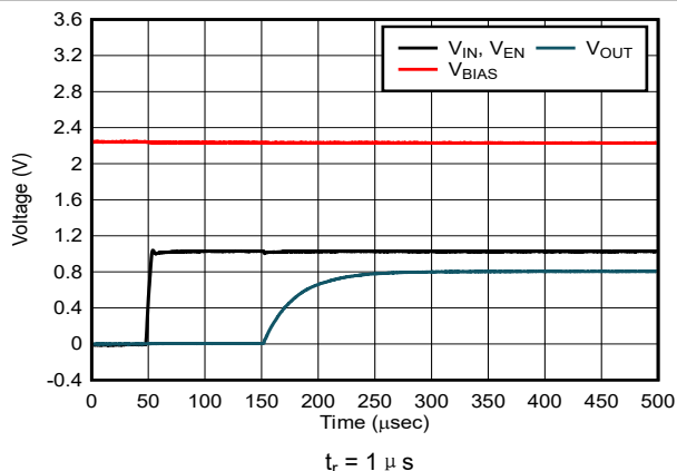
图 5-14. 在先施加 V_{\text{BIAS}} 后施加 V_{\text{IN}} 的情况下启动
