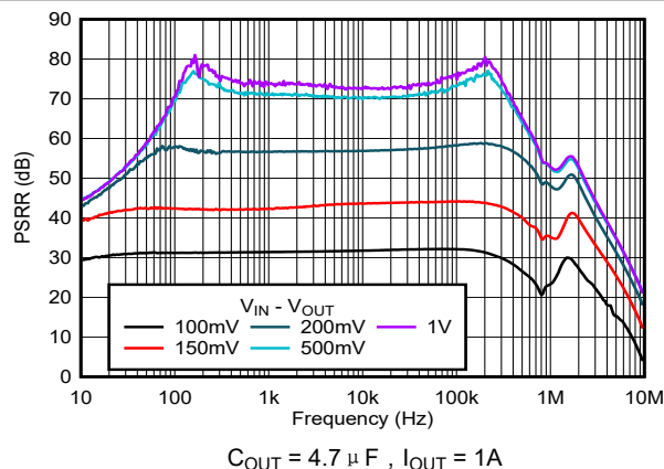
图 5-25. PSRR 与频率和 V_{\text{IN}} - V_{\text{OUT}} 间的关系
