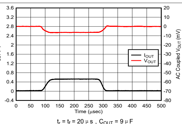
图 5-24. 从 10mA 至 500mA 的负载瞬态
