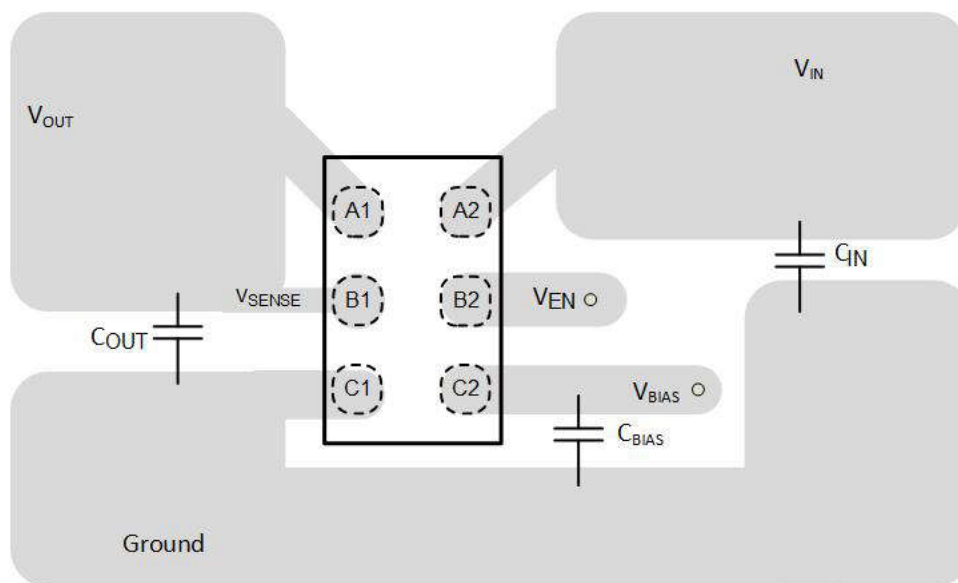
图 7-6. 建议布局 (YBK 封装)
