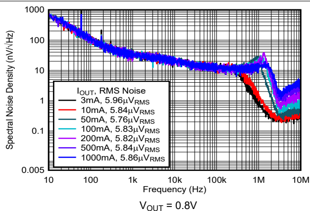
图 5-30. 输出噪声与频率和 I_{\text{OUT}} 间的关系
