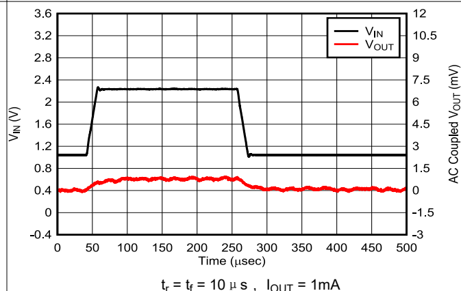
图 5-18. 从 1V 至 2.2V 的线路瞬态
