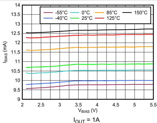
图 5-7. V_{\text{BIAS}} 输入电流与 V_{\text{BIAS}} 间的关系
