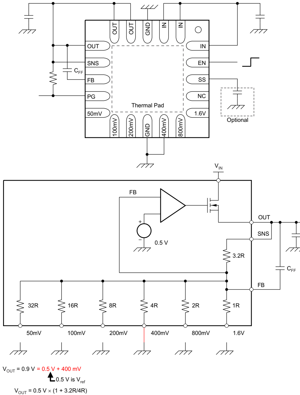
图 6-1. 0.9-V Configuration
