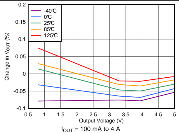
图 28. Load Regulation vs Output Voltage
