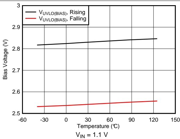
图 41. V_{BIAS} UVLO vs Temperature
