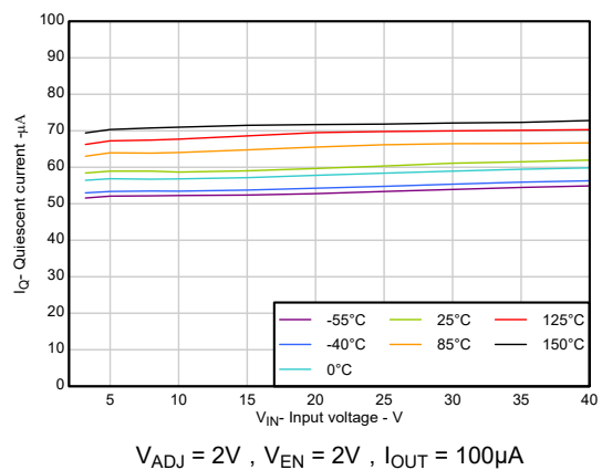
图 5-10. 静态电流与输入电压间的关系
