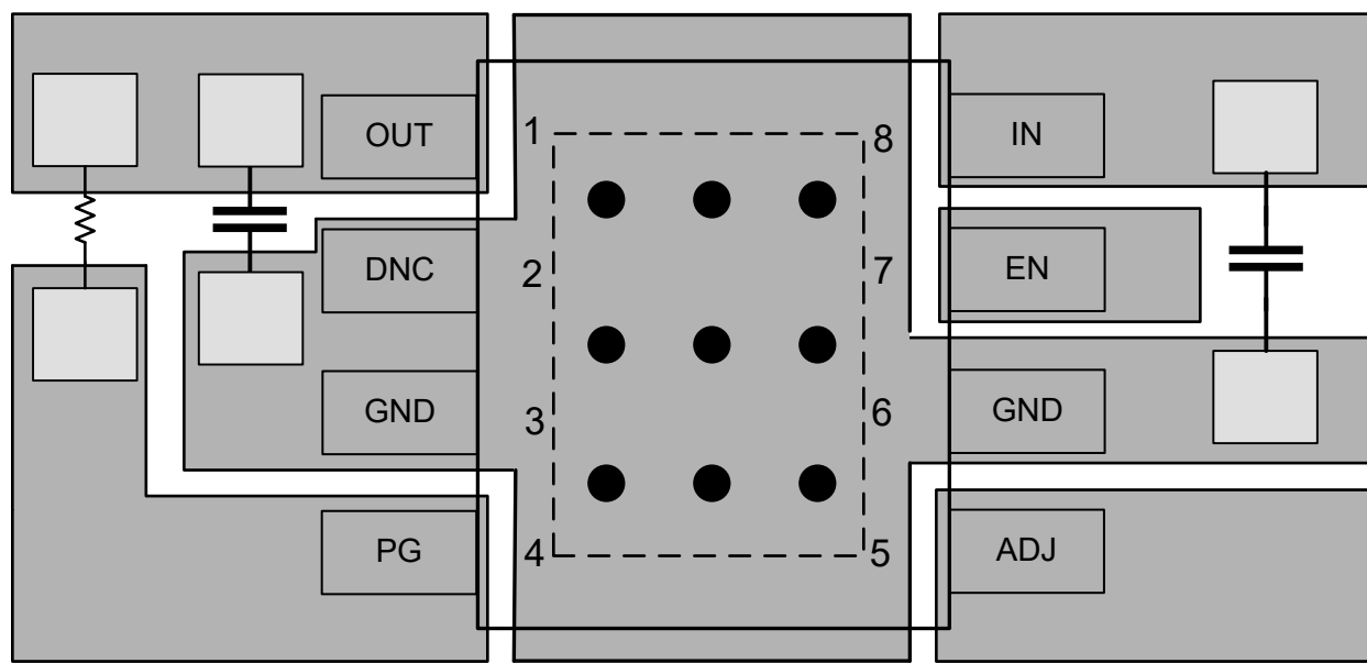
图 7-7. 布局示例
