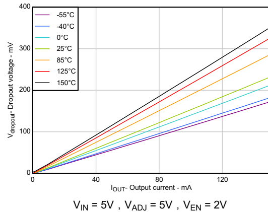
图 5-8. 压降电压与负载电流间的关系
