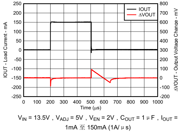
图 5-33. 负载瞬态
