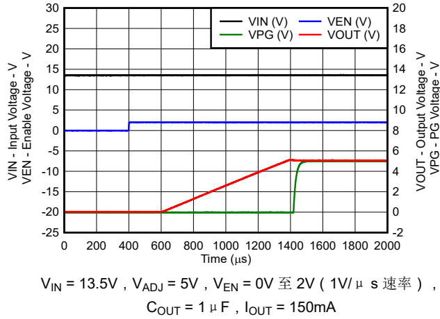
图 5-31. 启动曲线
