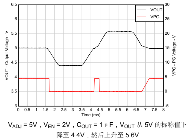
图 5-34. 电源正常状态指示功能
