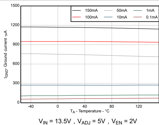
图 5-11. 接地电流与环境温度间的关系
