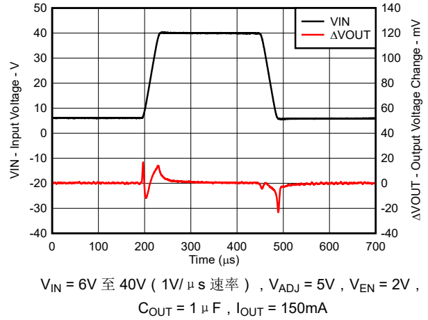
图 5-32. 线路瞬态
