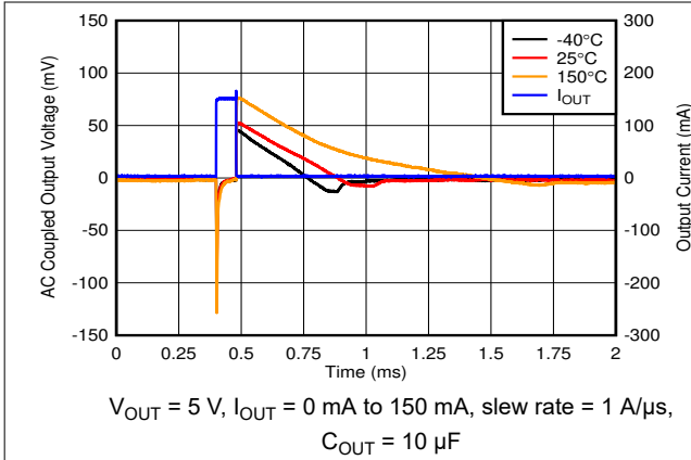
图 6-19. Load Transient, No Load to 150-mA
