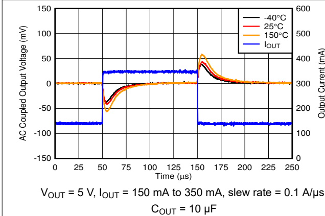
图 6-21. Load Transient, 150-mA to 350-mA
