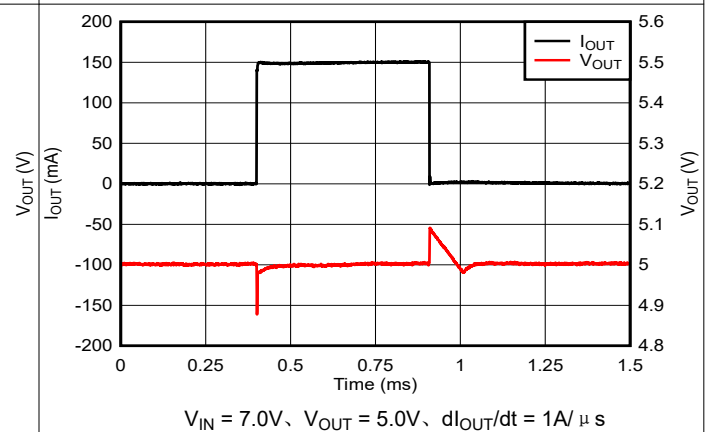
图 5-30. 负载瞬态 (1mA 至 150mA)
