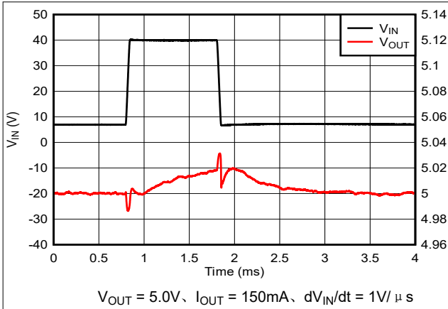
图 5-25. V_{IN} 线路瞬态 (7V 至 40V)
