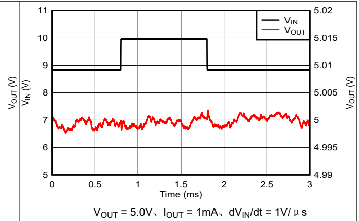
图 5-26. V_{IN} 线路瞬态 (8.8V 至 10V)
