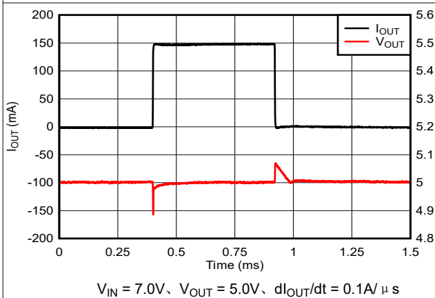
图 5-29. 负载瞬态 (1mA 至 150mA)
