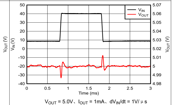
图 5-28. V_{IN} 线路瞬态 (8.8V 至 40V)
