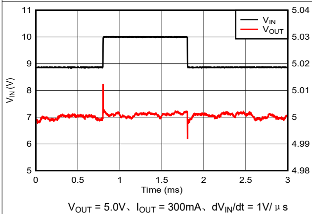
图 5-27. V_{IN} 线路瞬态 (8.8V 至 10V)
