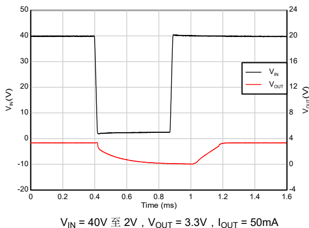
图 7-15. 欠压恢复 (40V 至 2V)
