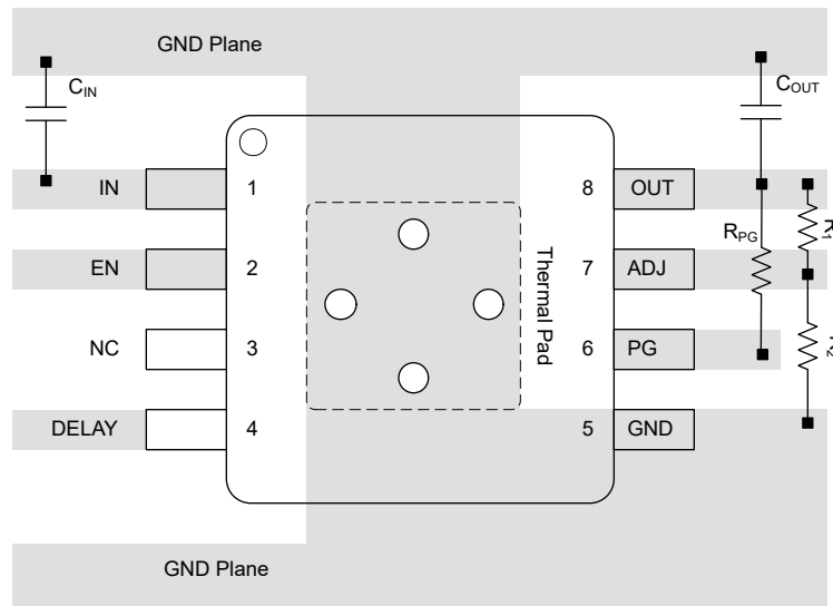
图 7-16. TPS7E66-Q1 DGN 封装的布局示例
