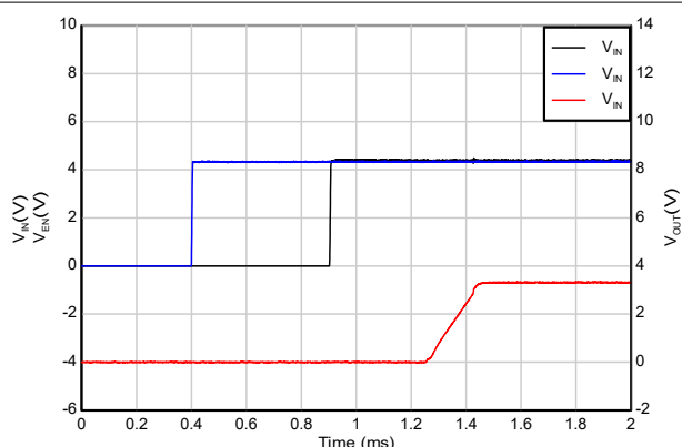
图 5-38. 时序启动 ( V_{IN} 在 EN 之后)
