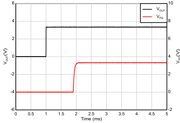
图 5-41. C_{DELAY} = 1\text{nF} 时的 PG 延迟
