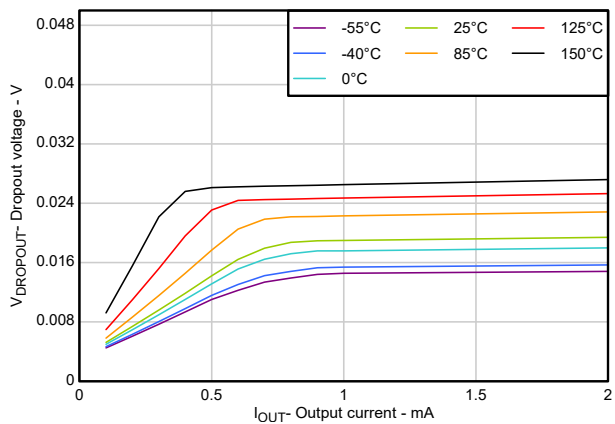
图 5-6. V_{DO} 与 I_{OUT} (mA) 间的关系
