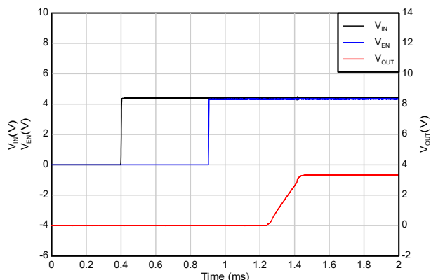
图 5-36. 时序启动 (EN 在 V_{IN} 之后)
