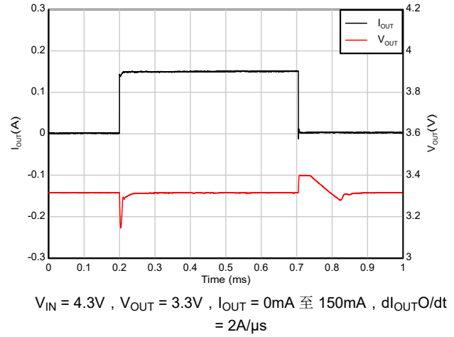
图 7-10. 负载瞬态 (0mA 至 150mA)
