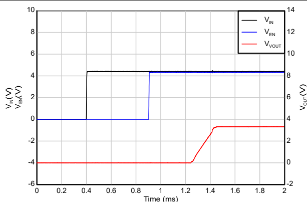
图 5-35. 时序启动 (EN 在 V_{IN} 之后)
