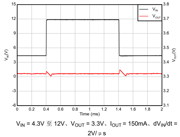
图 5-44. 线路瞬态 (4.3V 至 12V)
