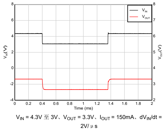
图 5-50. 压降恢复 (4.3V 至 3V)
