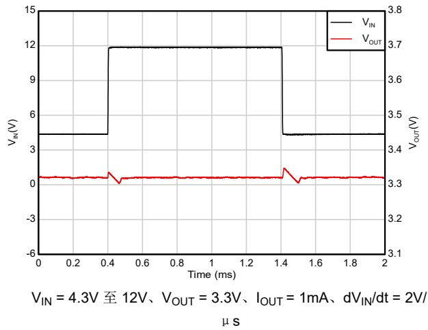
图 5-43. 线路瞬态 (4.3V 至 12V)
