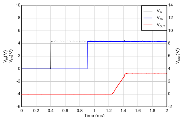
图 5-35. 时序启动 (EN 在 V_{IN} 之后)
