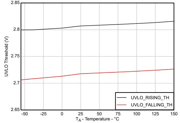
图 5-14. UVLO 阈值 ( V_{UVLO+}/V_{UVLO-} ) 与温度间的关系
