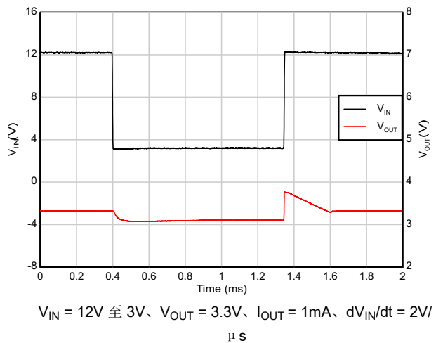
图 5-51. 压降恢复 (12V 至 3V)
