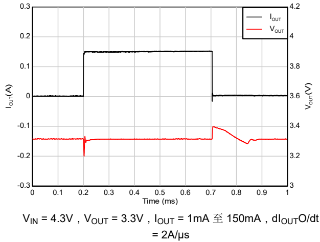
图 7-11. 负载瞬态 (1mA 至 150mA)
