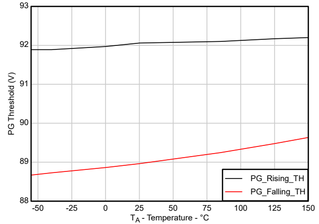
图 5-18. PG 阈值 ( V_{IT+(PG)}/V_{IT-(PG)} ) 与温度间的关系
