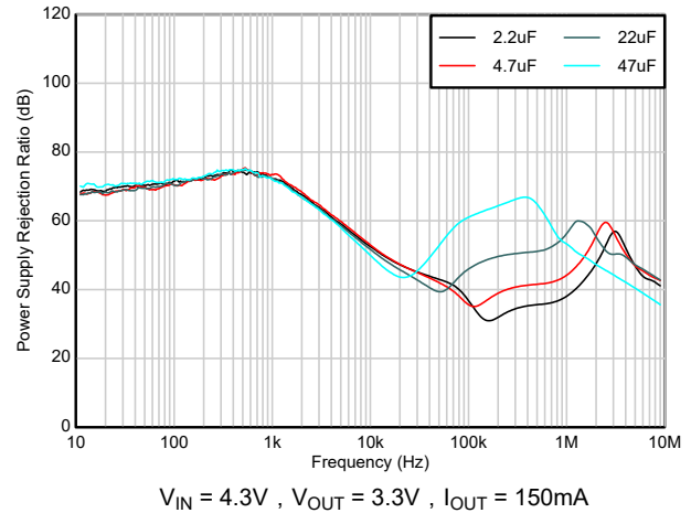
图 5-24. PSRR 与 C_{OUT} 间的关系
