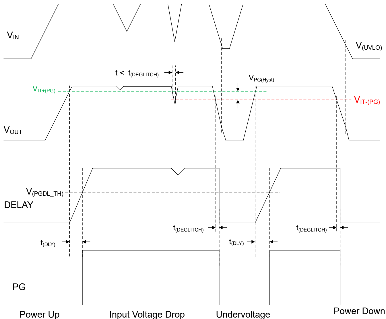
图 6-3. 典型的电源正常时序图
