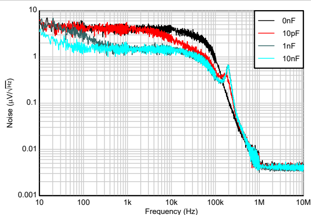
图 5-29. 噪声与 C_{FF} 间的关系
