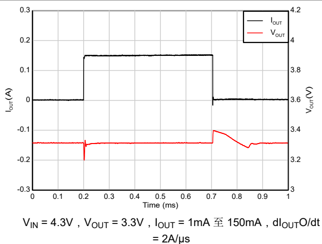
图 5-48. 负载瞬态 (1mA 至 150mA)
