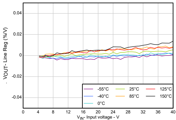
图 5-4. 线性调整率
