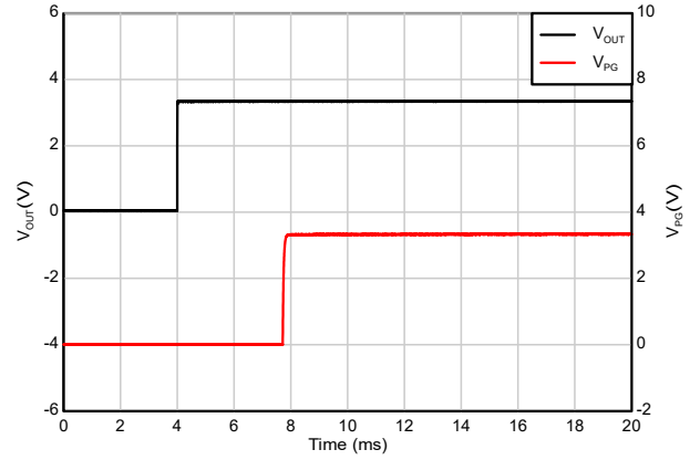
图 5-42. C_{DELAY} = 4.7\text{nF} 时的 PG 延迟
