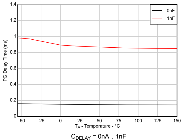
图 5-19. PG 延迟时间与温度间的关系
