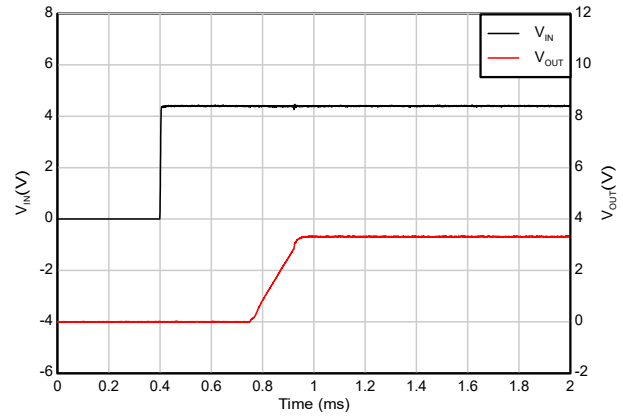
图 7-6. EN 与 V_{IN} 引脚短接启动
