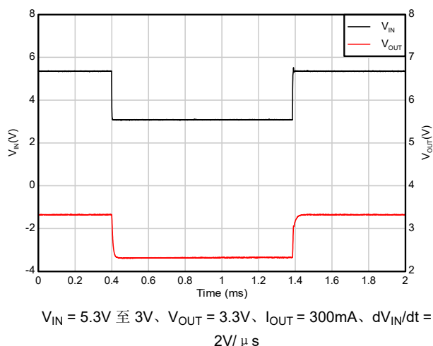
图 7-13. 压降恢复 (5.3V 至 3V)
