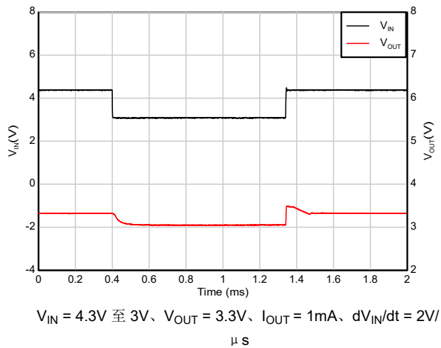
图 5-49. 压降恢复 (4.3V 至 3V)
