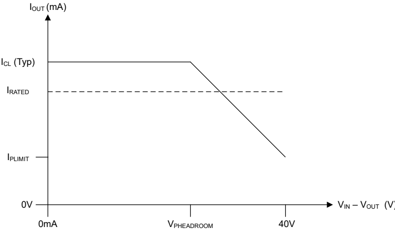
图 6-5. 功率限制
