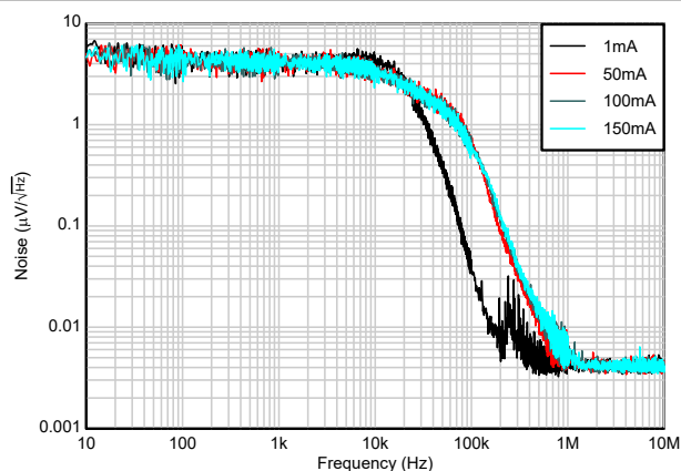
图 5-26. 噪声与 I_{OUT} 间的关系
