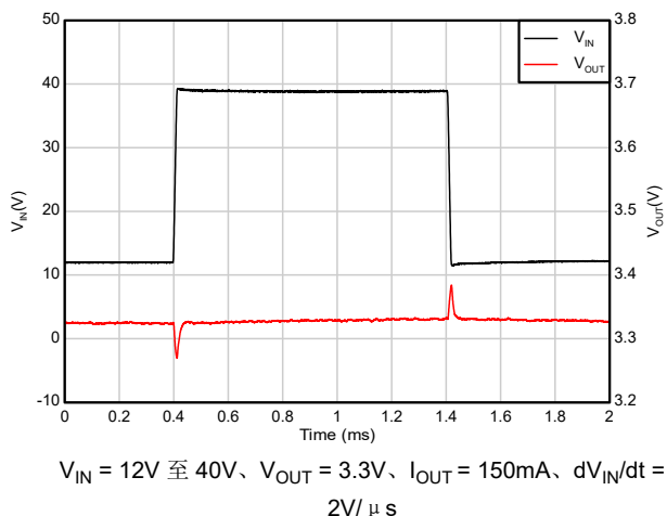
图 5-46. 线路瞬态 (12V 至 40V)
