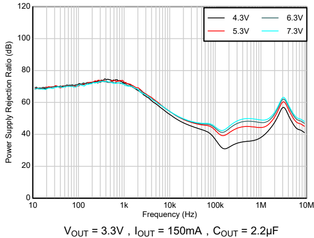
图 5-23. PSRR 与 V_{IN} 间的关系
