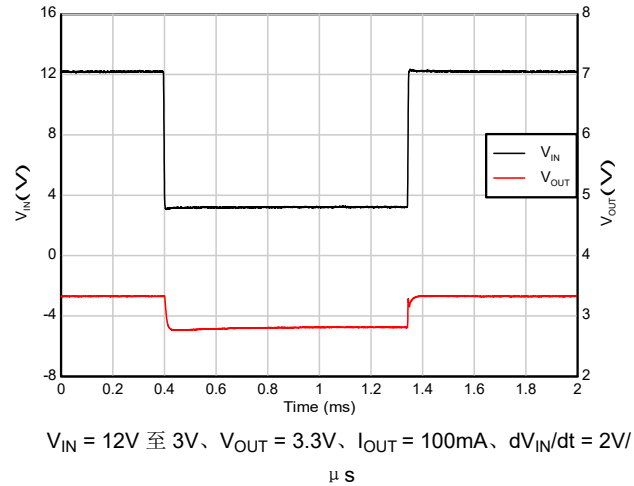
图 7-12. 压降恢复 (12V 至 3V)
