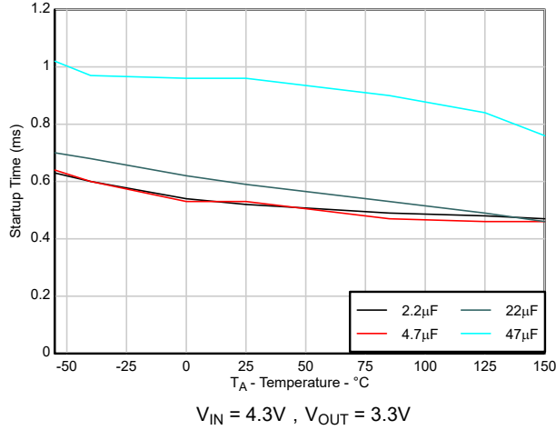
图 5-21. 启动时间与 C_{OUT} 间的关系
