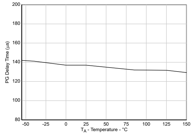
图 5-20. PG 抗尖峰脉冲时间与温度间的关系
