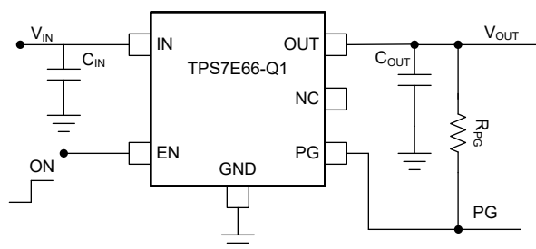
图 7-3. 典型应用电路（固定电压版本）
