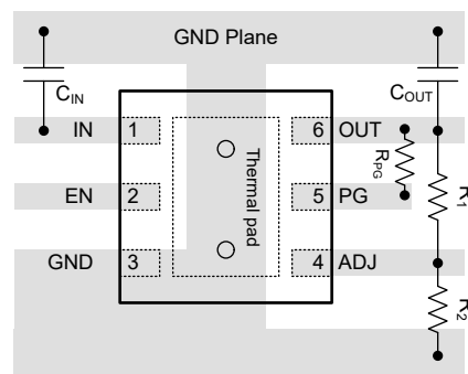
图 7-17. TPS7E66-Q1 DRV 封装的布局示例
