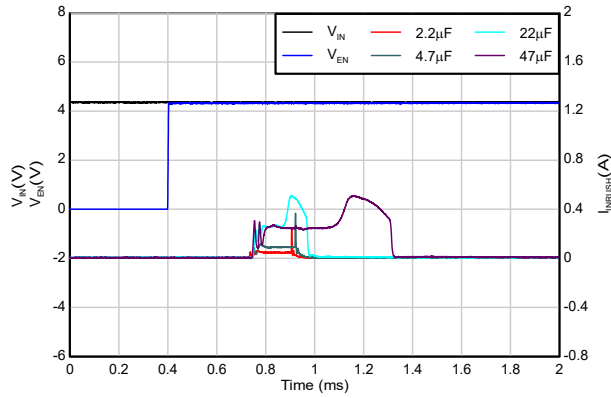
图 7-5. 浪涌电流与 C_{OUT} 间的关系
