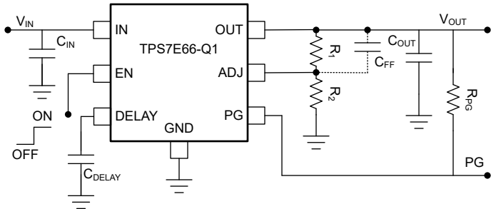
图 7-4. 典型应用电路 ( 可调电压版本 )
