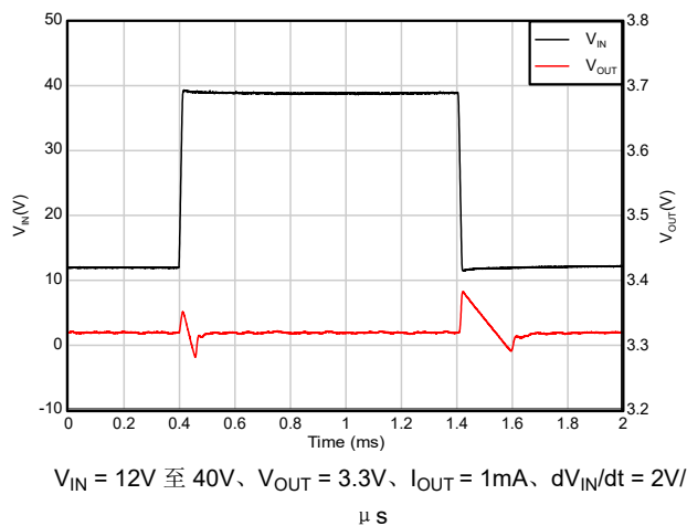
图 5-45. 线路瞬态 (12V 至 40V)
