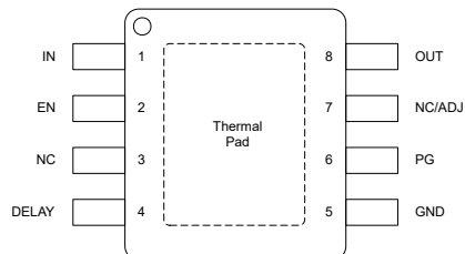
图 4-3. DGN 封装 (固定/ADJ), 8-引脚 HVSSOP (顶视图)
