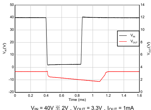
图 7-14. 欠压恢复 (40V 至 2V)
