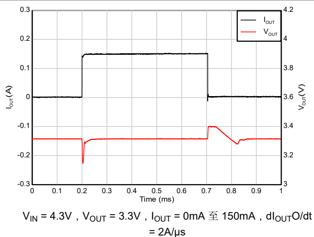
图 5-47. 负载瞬态 (0mA 至 150mA)
