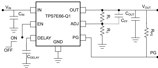
典型应用
