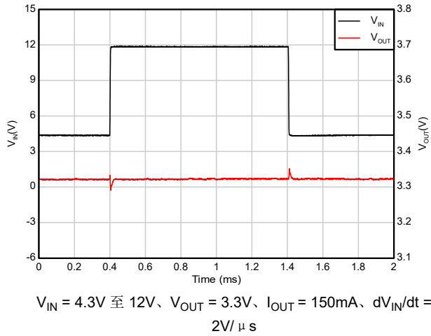
图 7-9. 线路瞬态 (4.3V 至 12V)
