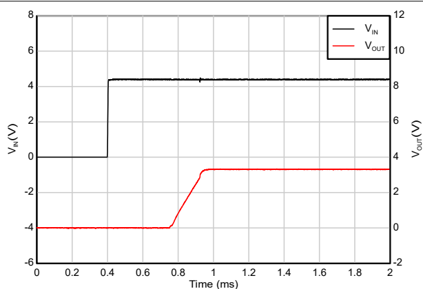
图 5-32. EN 与 V_{IN} 引脚短接启动
