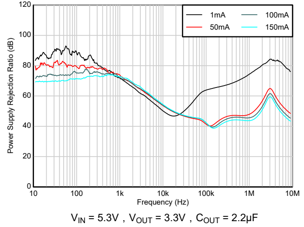
图 5-22. PSRR 与 I_{OUT} 间的关系
