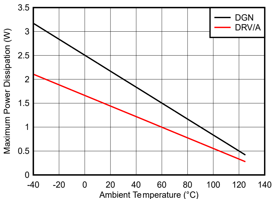
图 7-2. TPS7E66-Q1 允许的功率耗散
