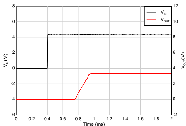
图 5-30. 启动与 C_{OUT} 间的关系
