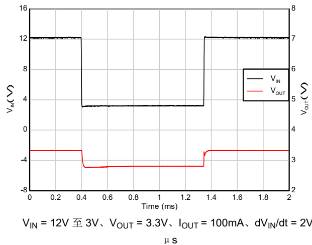
图 5-52. 压降恢复 (12V 至 3V)
