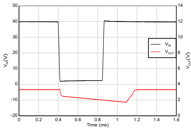
图 5-52. 欠压恢复 (40V 至 2V)
