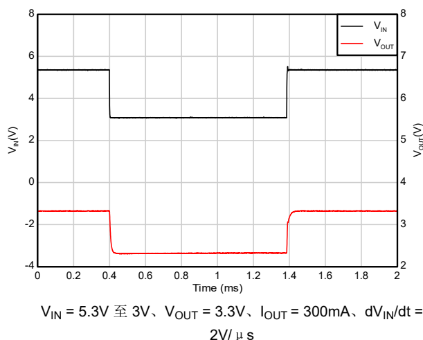
图 7-13. 压降恢复 (5.3V 至 3V)
