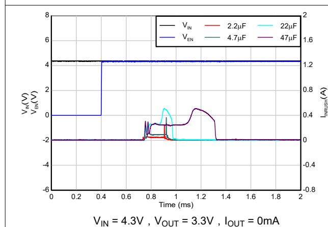
图 5-31. 浪涌电流与 C_{OUT} 间的关系
