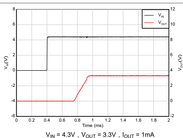
图 5-32. EN 与 V_{IN} 引脚短接启动
