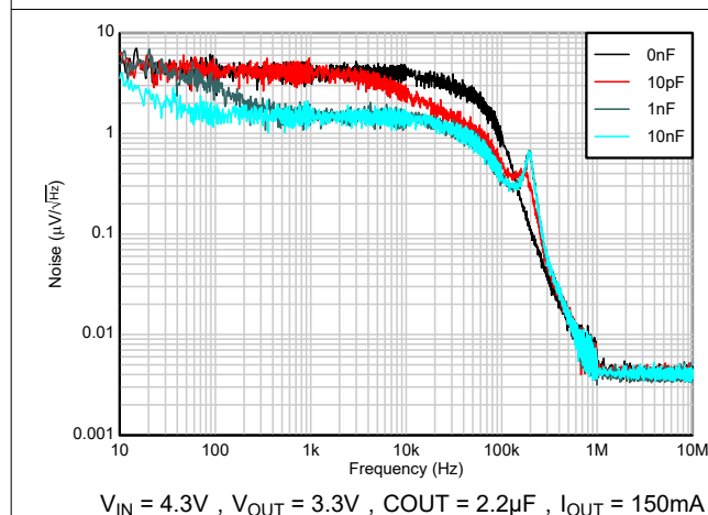
图 5-29. 噪声与 C_{FF} 间的关系
