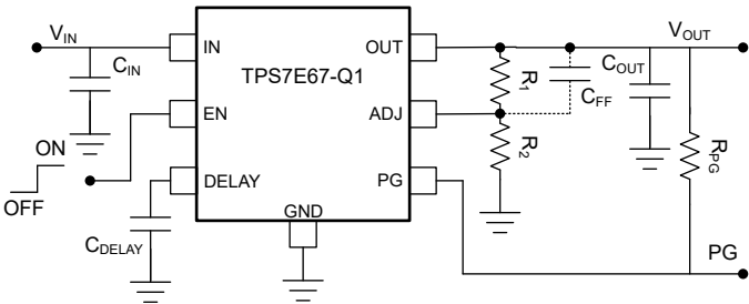
图 7-4. TPS7E67-Q1 可调节 LDO 稳压器编程
