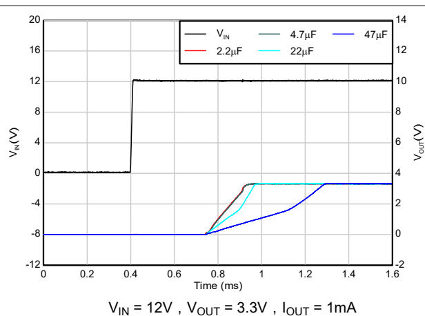
图 5-30. 启动与 C_{OUT} 间的关系
