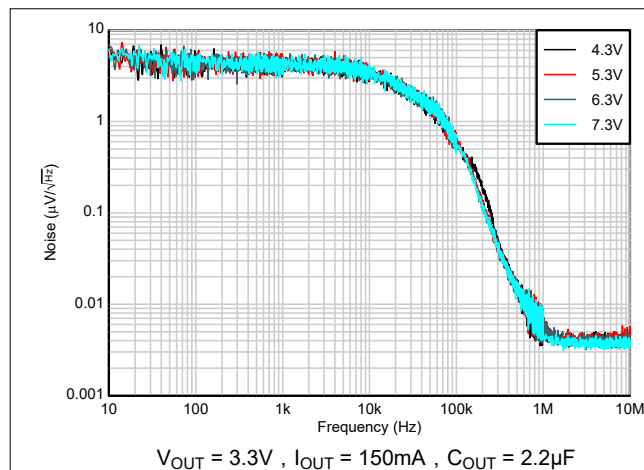
图 5-27. 噪声与 V_{IN} 间的关系
