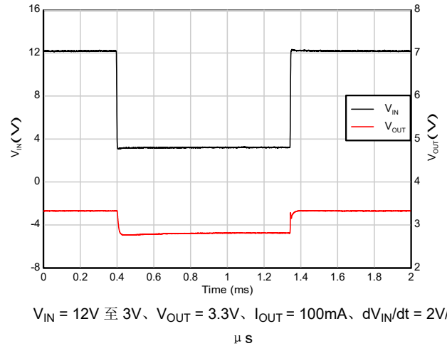
图 7-12. 压降恢复 (12V 至 3V)
