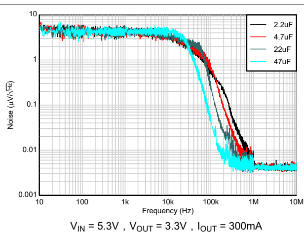
图 5-28. 噪声与 C_{OUT} 间的关系
