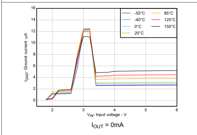
图 5-11. 接地电流与输入电压间的关系
