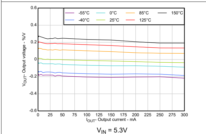
图 5-5. 精度与输出电流之间的关系
