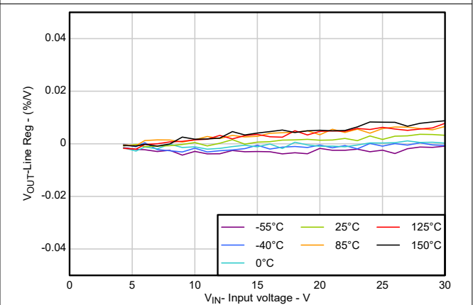
图 5-6. 线性调整率与输入电压间的关系
