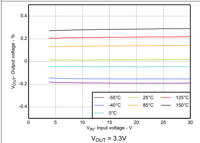
图 5-3. 精度与输入电压之间的关系
