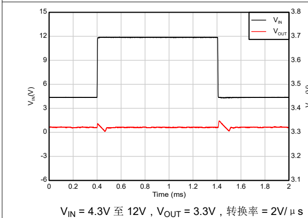
图 5-29. 线路瞬态
