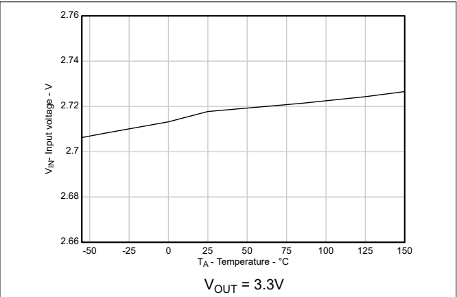
图 5-2. 下降输入电源 UVLO 与温度之间的关系
