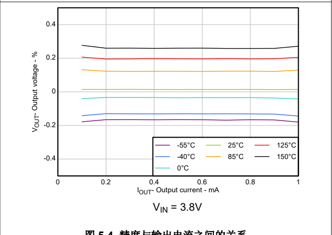
图 5-4. 精度与输出电流之间的关系
