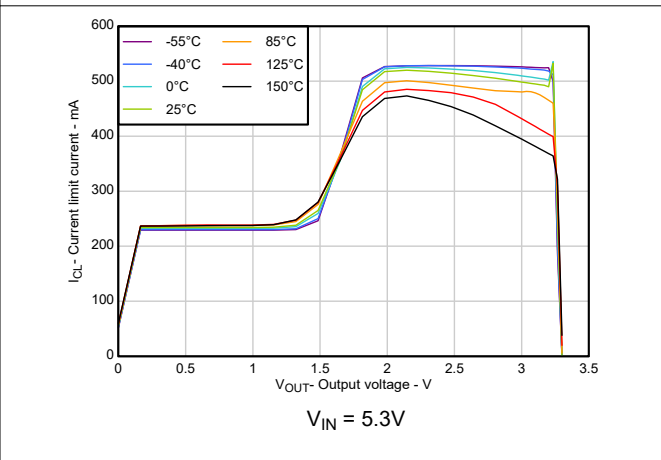
图 5-10. 电流限制与输出电压间的关系
