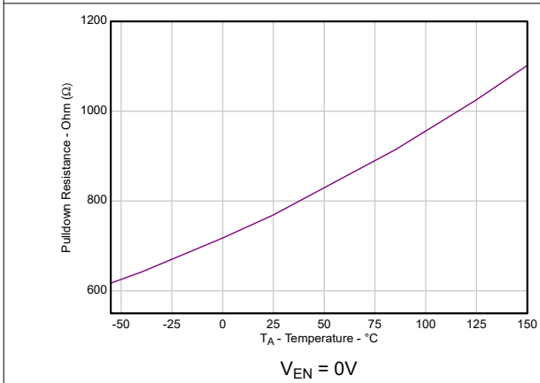
图 5-27. 输出放电电阻与温度之间的关系
