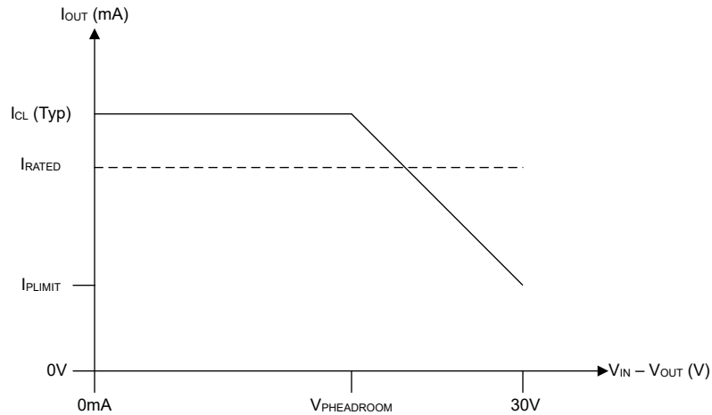
图 6-4. 功率限制
