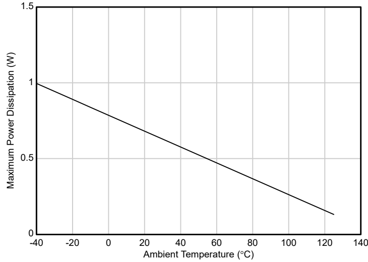
图 7-2. TPS7E72 (DBV) 允许的功率耗散
