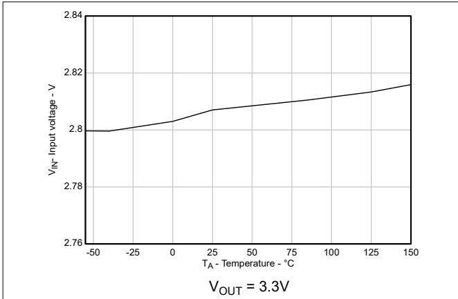
图 5-1. 上升输入电源 UVLO 与温度之间的关系
