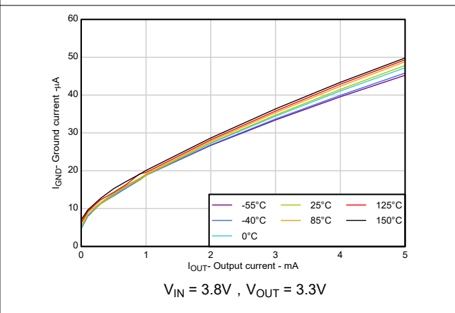
图 5-12. 接地电流与输出电流间的关系
