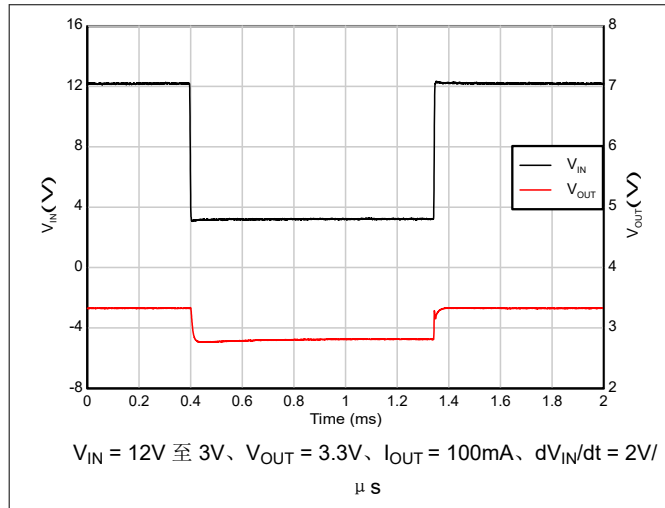
图 5-49. 压降恢复 (12V 至 3V)
