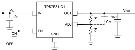
图 3-1. 典型应用
