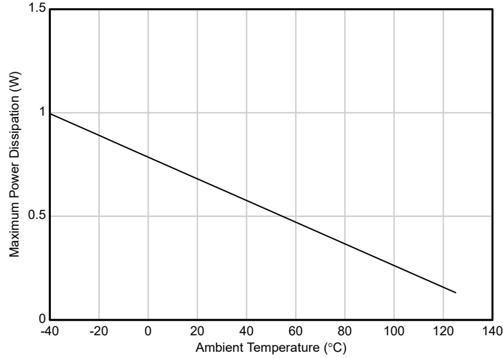
图 7-2. TPS7E81-Q1 (DBV) 允许的功率耗散
