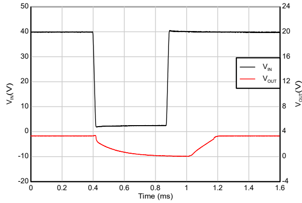
图 5-53. 欠压恢复 (40V 至 2V)
