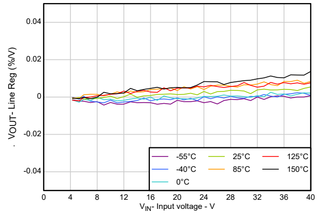
图 5-4. 线性调整率
