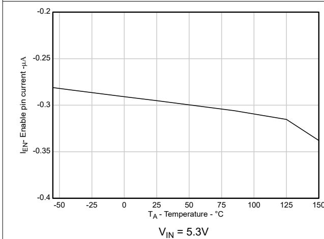
图 5-15. EN 泄漏电流 I_{EN} 与温度间的关系
