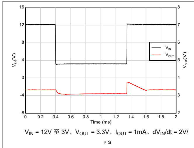
图 5-45. 压降恢复 (12V 至 3V)
