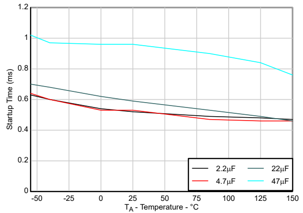
图 5-20. 启动时间与 C_{\text{OUT}} 间的关系
