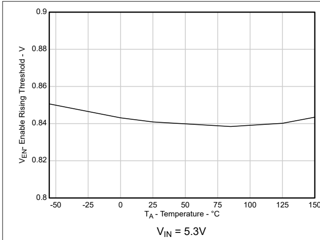
图 5-13. EN 上升阈值电压 V_{IH(EN)} 与温度间的关系
