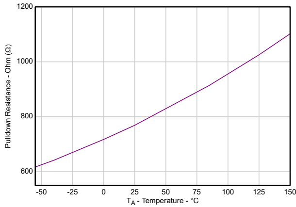
图 5-17. 输出端的下拉电阻 ( R_{\text{Discharge}} ) 与温度间的关系
