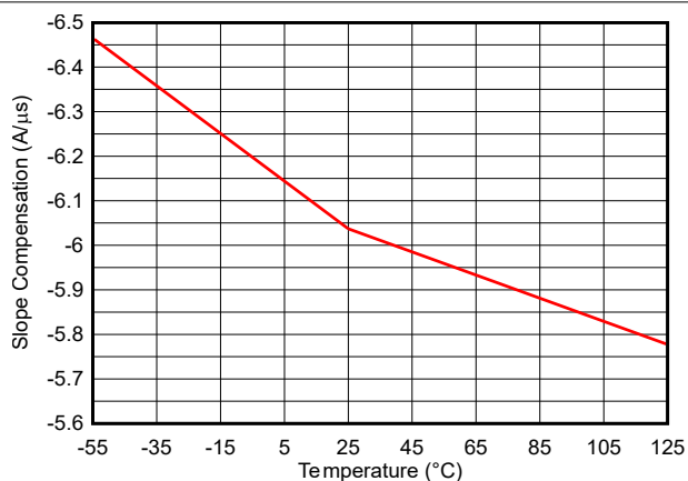
图 7-40. 100kHz 下斜率补偿与温度间的关系
