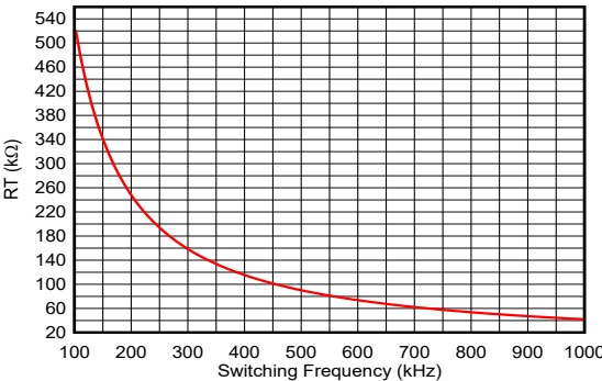
图 9-4. 标称 RT 与开关频率间的关系
