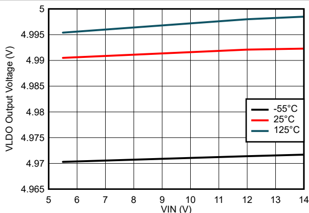
图 6-2. 内部线性稳压器输出电压与输入电压间的关系
