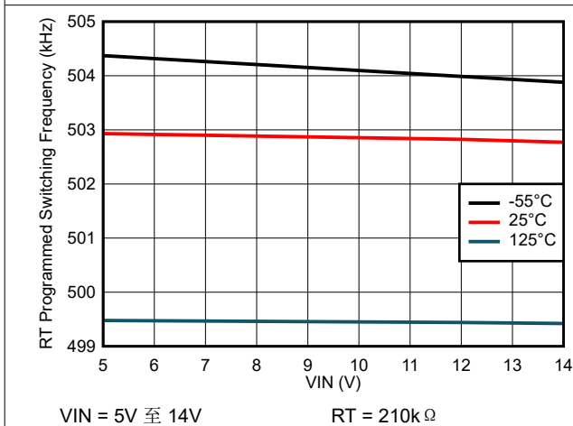
图 6-17. 开关频率与输入电压间的关系
