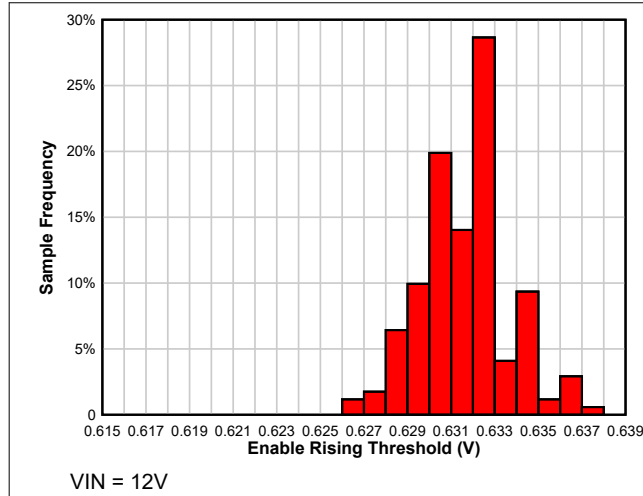
图 6-43. T_A = 125^\circ\text{C} 时的使能上升阈值分布
