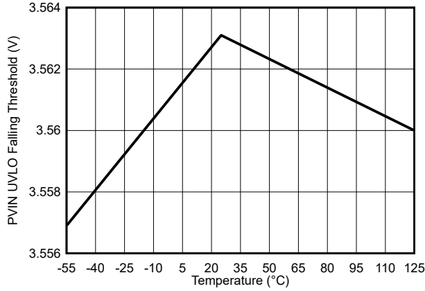
图 6-7. PVIN UVLO 下降阈值与温度间的关系
