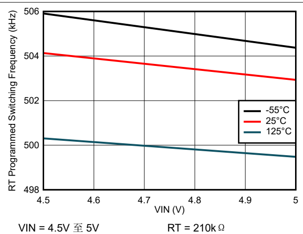
图 6-16. 开关频率与输入电压间的关系
