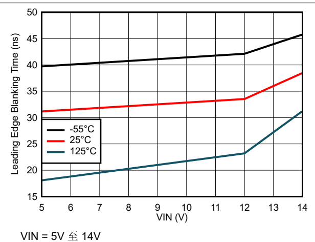
图 6-38. 前沿消隐时间与输入电压间的关系
