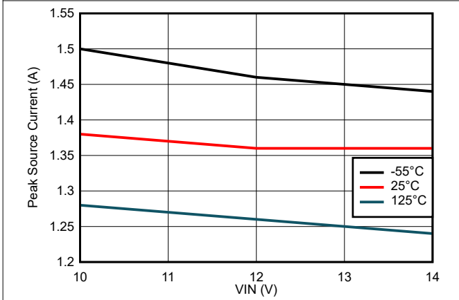
图 7-9. Peak Source Current vs VIN Voltage
