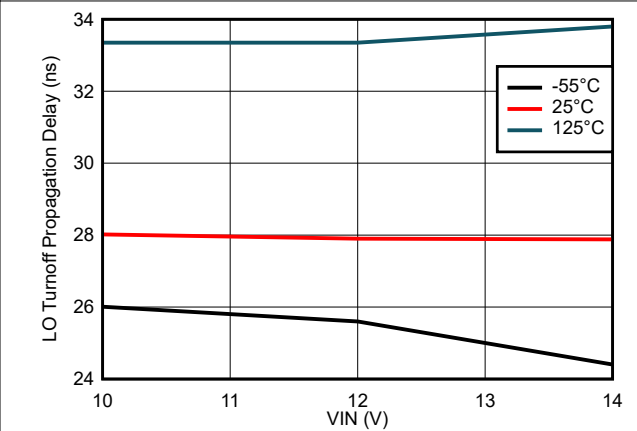
图 7-4. LO Turnoff Propagation Delay vs VIN Voltage (IIM)
