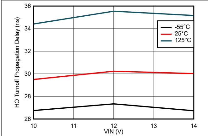
图 7-7. HO Turnoff Propagation Delay vs VIN Voltage (IIM)
