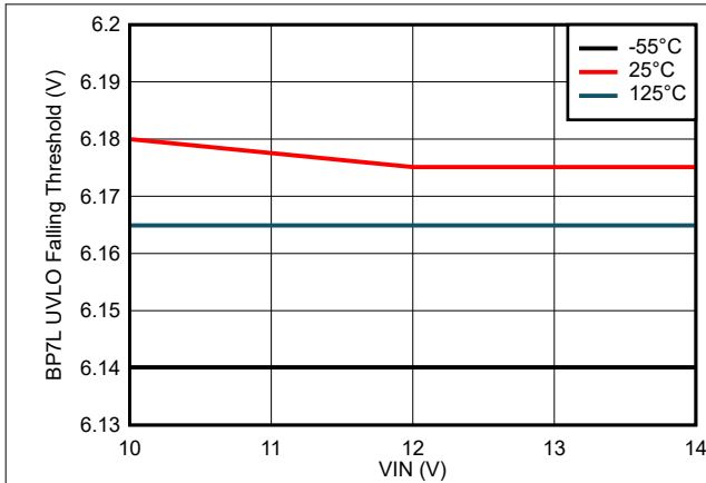
图 7-25. BP7L UVLO Falling Threshold vs VIN Voltage
