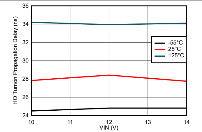
图 7-8. HO Turnon Propagation Delay vs VIN Voltage (IIM)
