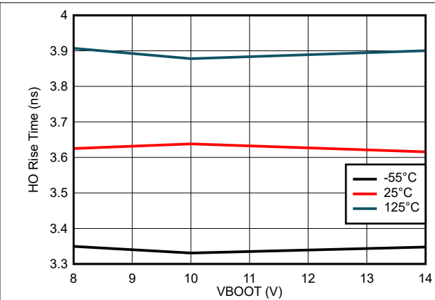
图 7-14. HO Output Rise Time vs BOOT Voltage
