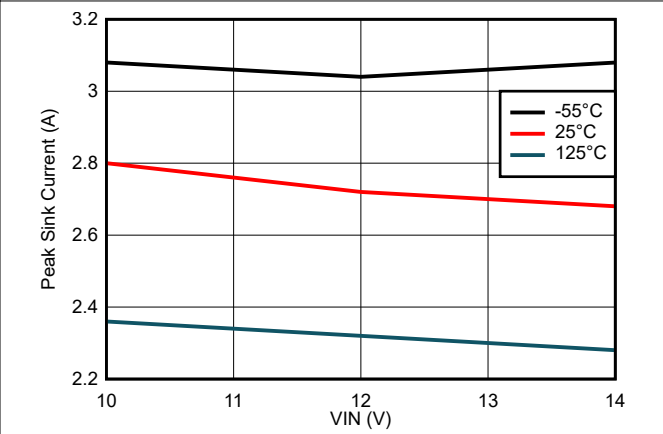
图 7-10. Peak Sink Current vs VIN Voltage
