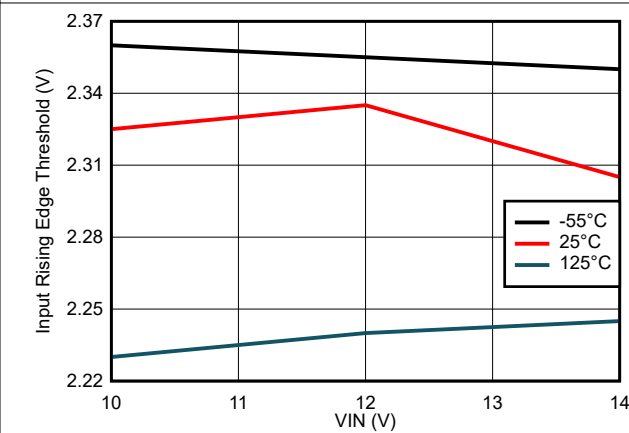
图 7-16. Input Rising Edge Threshold vs VIN Voltage
