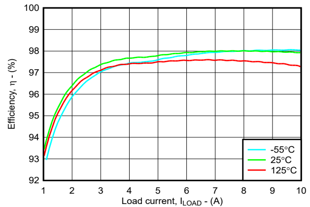
图 6-44. 100V 至 28V 效率
