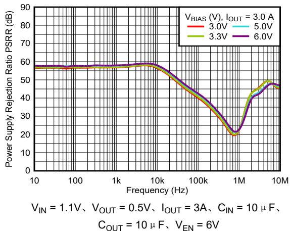
图 5-5. BIAS PSRR 与频率和 V_{BIAS} 间的关系
