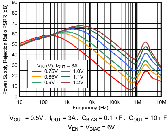
图 5-1. IN PSRR 与频率和 V_{IN} 间的关系
