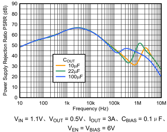
图 5-3. IN PSRR 与频率和 C_{OUT} 间的关系
