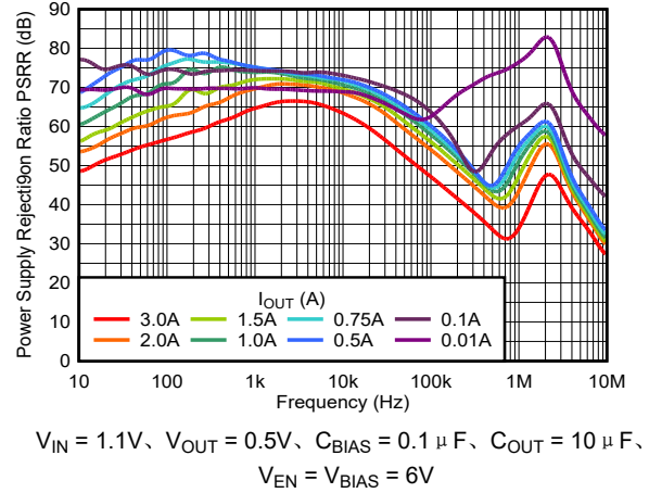
图 5-2. 在 V_{OUT} = 0.5\text{V} 时, IN PSRR 与频率和 I_{OUT} 间的关系
