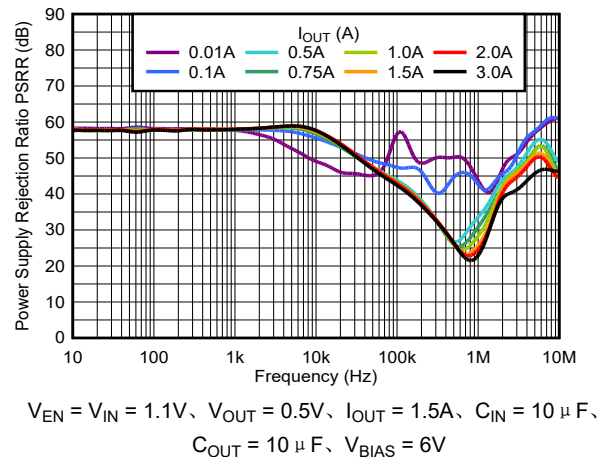
图 5-6. BIAS PSRR 与频率和 I_{OUT} 间的关系
