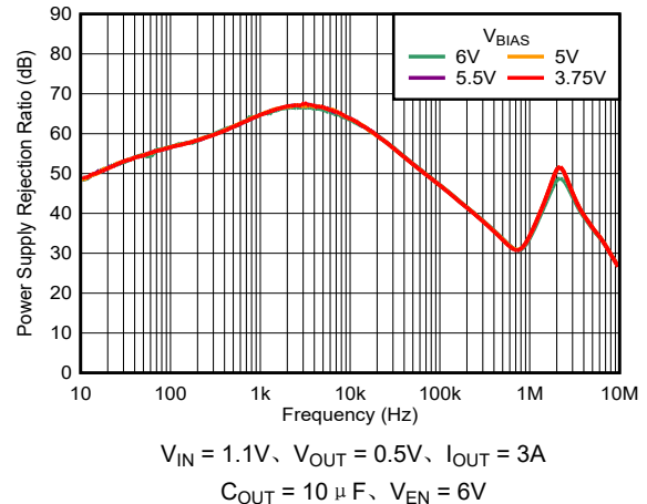
图 5-4. IN PSRR 与频率和 V_{BIAS} 间的关系
