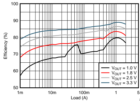
效率与输出电流, V_{IN}=12V
