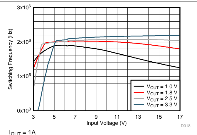
图 23. Switching Frequency
