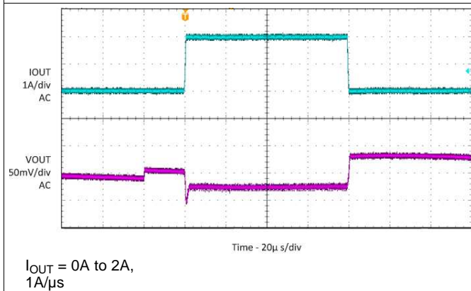
图 26. Load Transient
