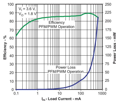
图 2. 效率与 负载电流间的关系
