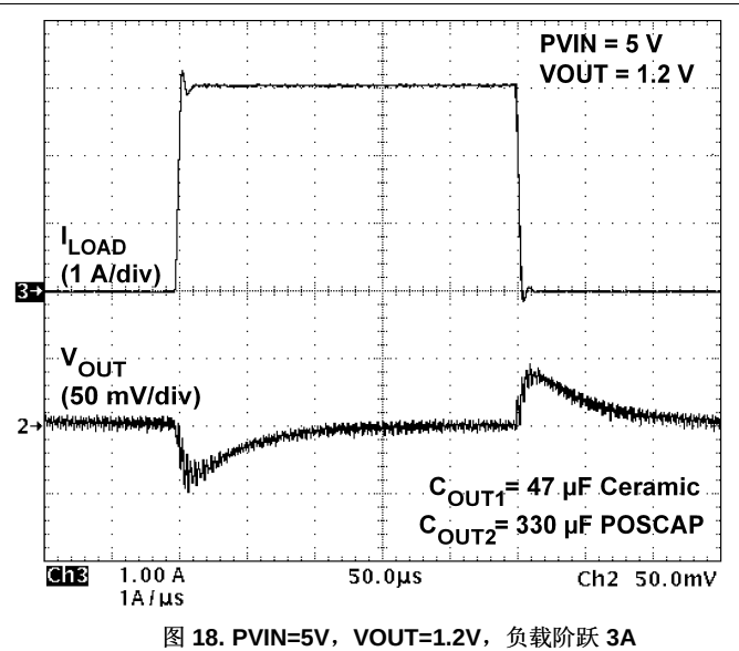
图 18. PV_{IN}=5V , V_{OUT}=1.2V , 负载阶跃 3A
