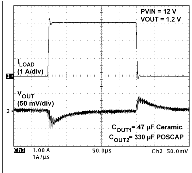
图 17. PV_{IN}=12V , V_{OUT}=1.2V , 负载阶跃 3A
