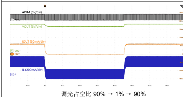
图 8-8. 调光瞬态
