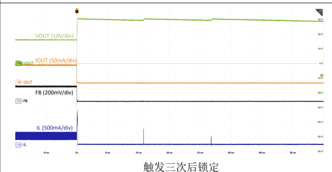
图 8-9. 开路 LED 过压保护
