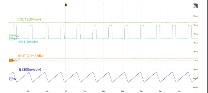
图 8-3. 开关调光占空比 = 10%
