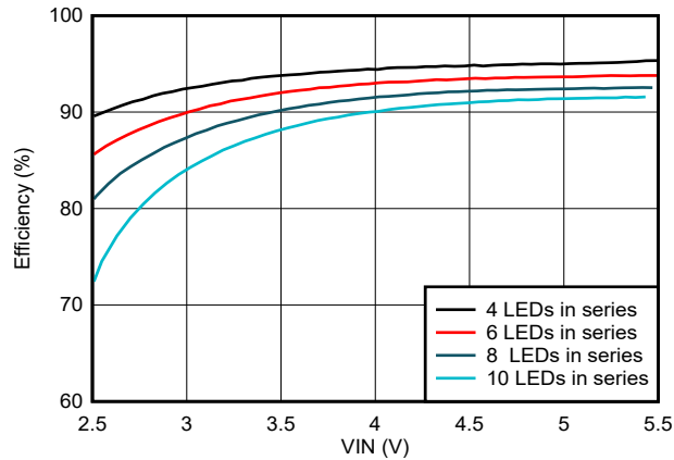
图 6-5. 效率与 VIN 间的关系
