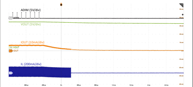
图 8-7. 关断调光占空比为 10%
