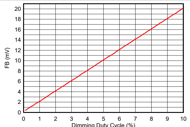
图 6-8. FB 与调光占空比 0.1%~10% 的关系
