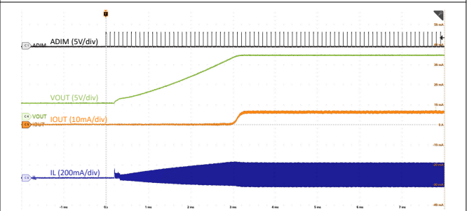
图 8-5. 启动调光占空比为 10%
