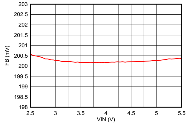
图 6-6. FB 与 VIN 间的关系
