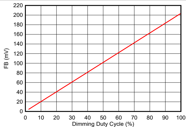
图 6-7. FB 与调光占空比 1%~100% 的关系
