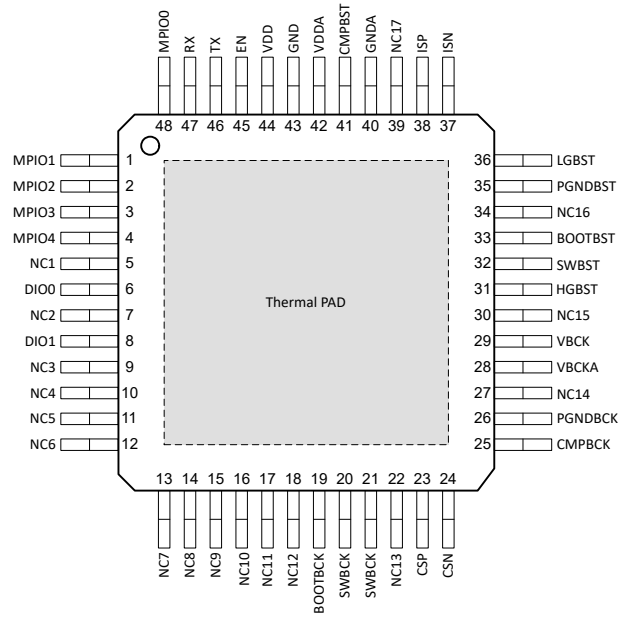
图 4-2. PHP 封装 48 引脚 HTQFP (底部外露焊盘) 顶视图
