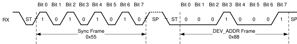
图 6-15. Synchronization Byte
