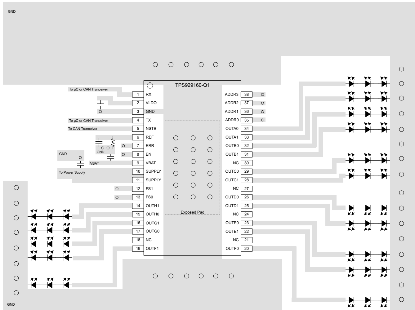
图 7-5. TPS929160-Q1 Layout
