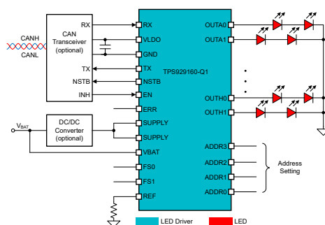
典型应用图
