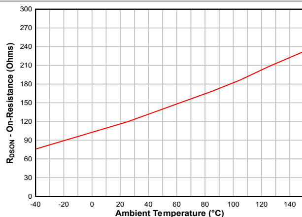
图 6-9. 典型导通电阻与环境温度间的关系
