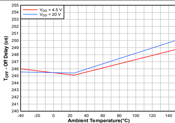
图 6-8. 输入到输出关闭延迟 ( V_{IN} = 1000\text{V} )
