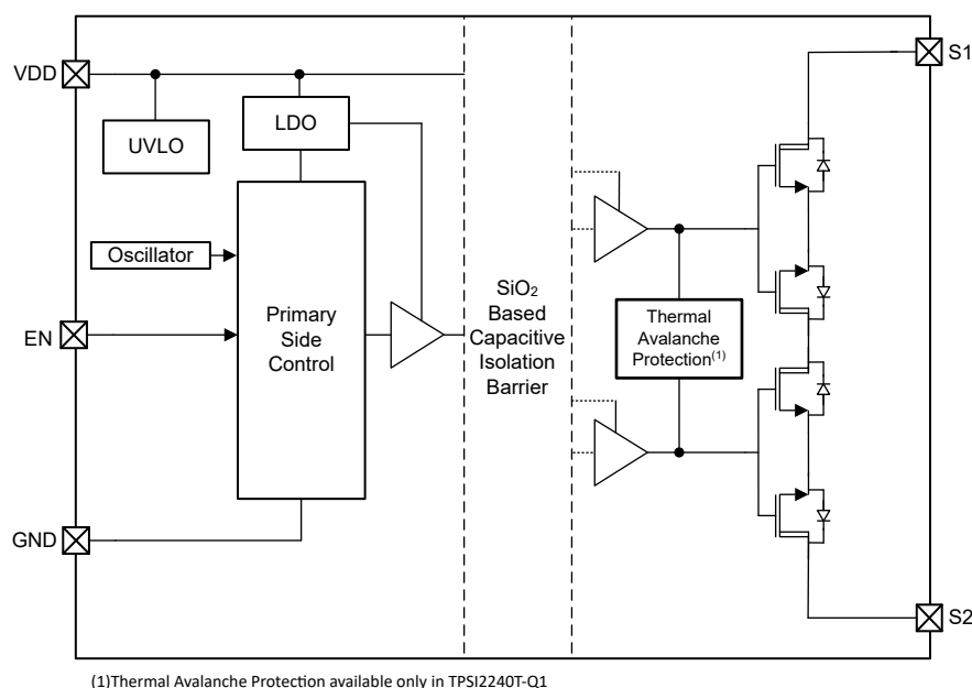
图 8-1. TPSI2240-Q1 方框图
