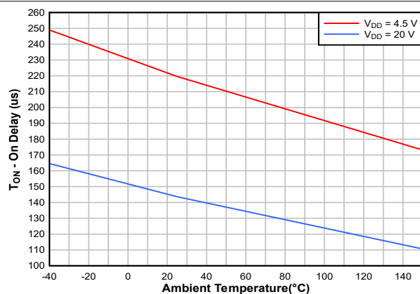
图 6-7. 输入到输出开启延迟 ( V_{IN} = 1000\text{V} )
