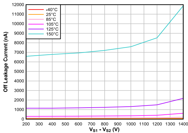
图 6-5. 关断泄漏电流与输出电压间的关系
