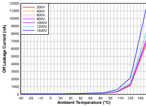
图 6-3. 关断泄漏电流与环境温度间的关系
