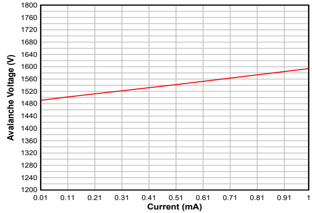
图 6-2. 雪崩电压与雪崩电流间的关系
