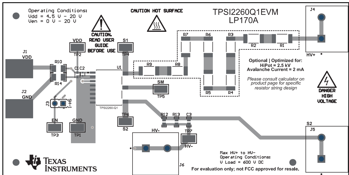
图 9-9. TPSI2260-Q1 EVM - 复合视图
