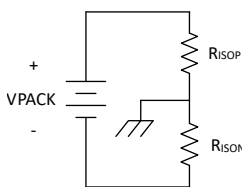
图 9-1. 绝缘电阻模型
