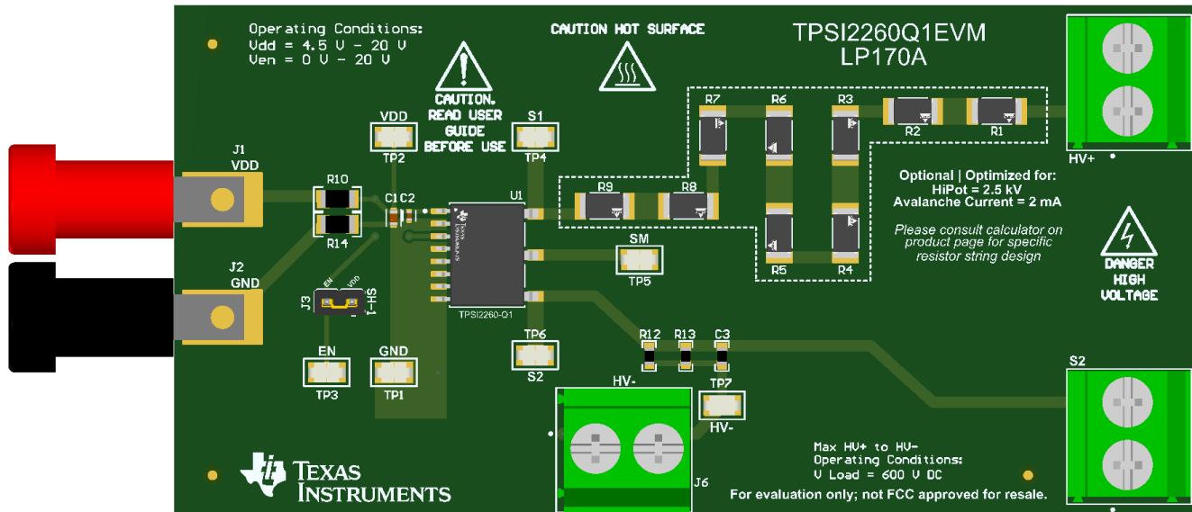
图 9-8. TPSI2260-Q1 EVM - 组件视图
