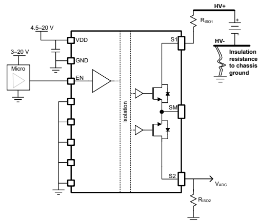
TPSI2260-Q1 简化版应用原理图
