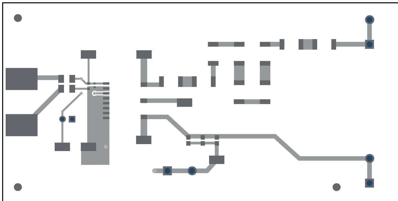
图 9-10. TPSI2260-Q1 EVM - 顶层
