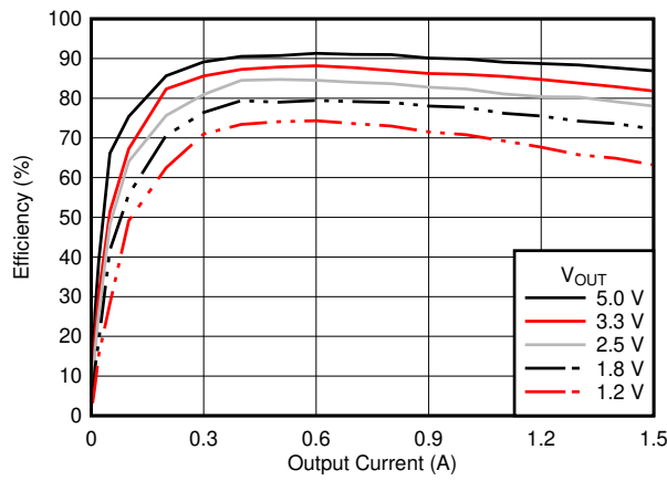
图 7-1. Efficiency
