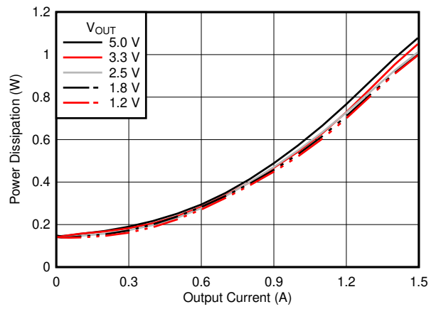
图 7-2. Power Dissipation
