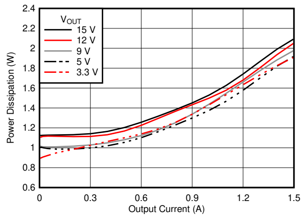
图 7-14. Power Dissipation
