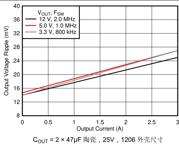
图 7-21. 输出电压纹波
