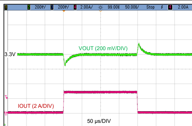
图 9-4. 负载瞬态 (0A 至 3A, 1A/μs)
