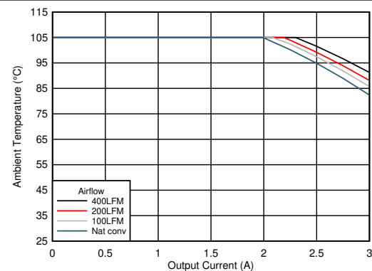
图 7-12. 安全工作区
