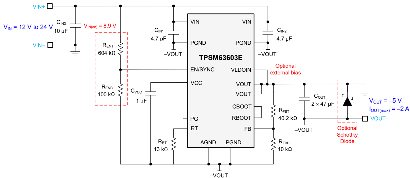
图 9-12. 电路原理图
