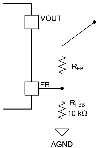
图 8-2. FB 电阻分压器
