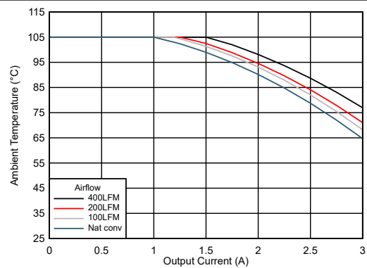
图 7-18. 安全工作区
