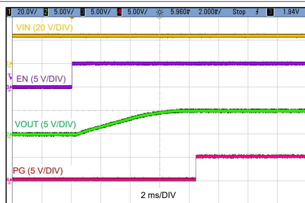
图 9-2. 启动波形
