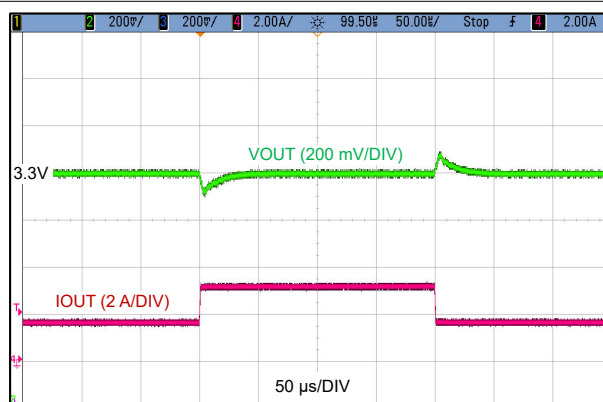
图 9-5. 负载瞬态 (1.5A 至 3A, 1A/μs)
