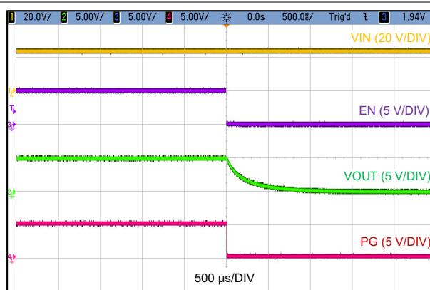
图 9-3. 关断波形
