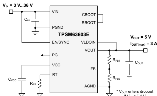
典型原理图
