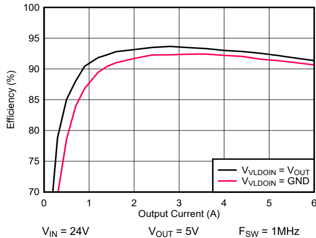
图 8-5. 通过外部偏置提高效率
