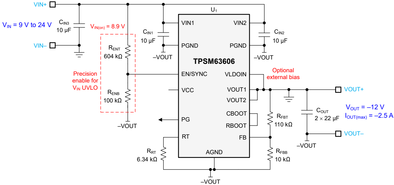
图 9-12. 电路原理图
