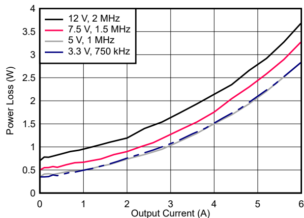
图 7-15. 功率损耗
