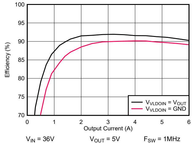
图 8-6. 通过外部偏置提高效率
