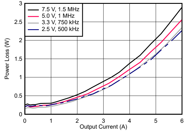
图 7-10. 功率损耗
