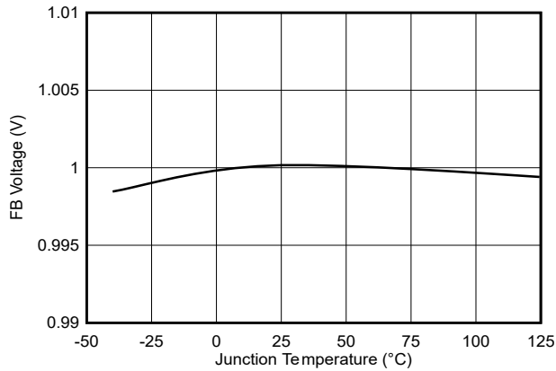
图 7-3. 反馈电压
