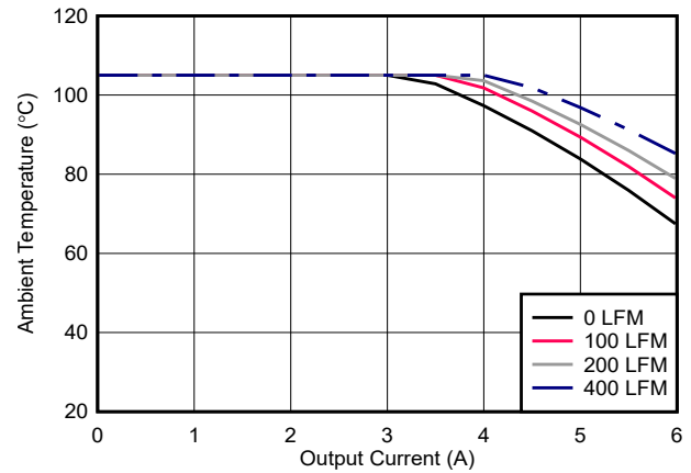
图 7-12. 安全工作区 ( V_{OUT} = 3.3V , F_{SW} = 750\text{kHz} )
