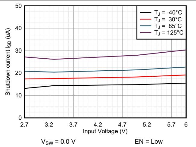
图 6-2. Shutdown Current
