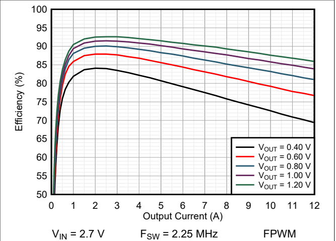
图 9-9. Efficiency TPSM8287A12BBS
