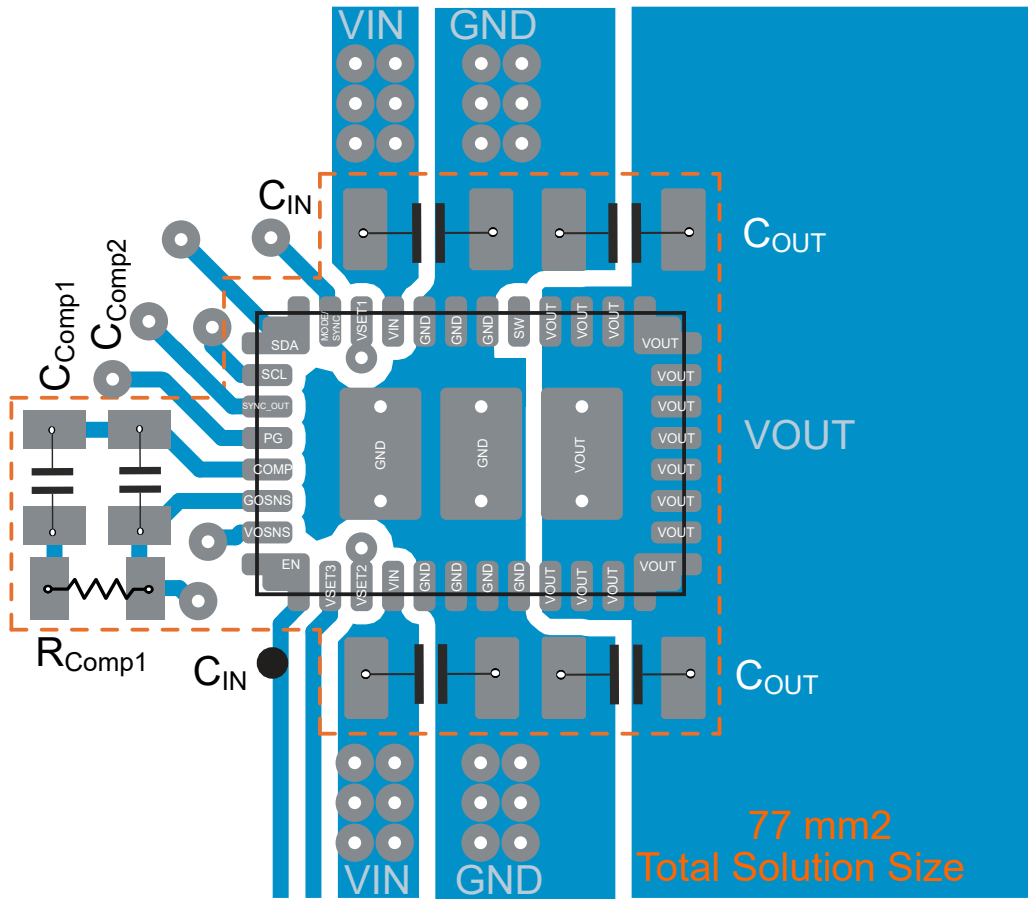
图 9-57. Layout Example
