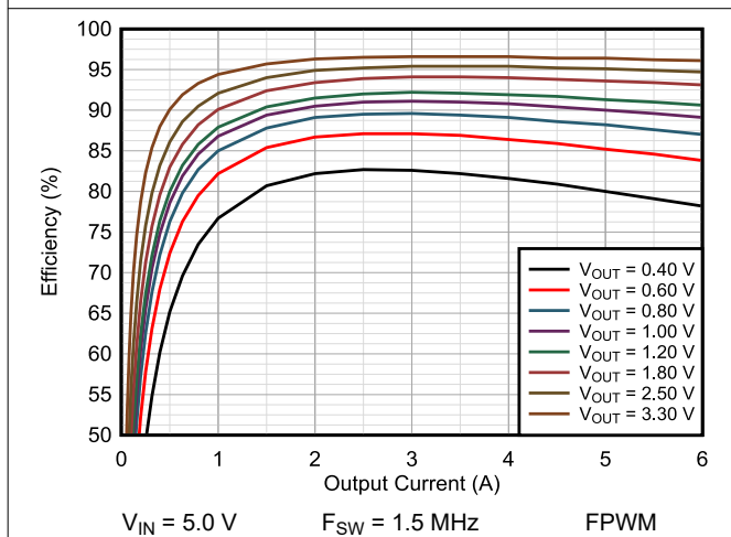
图 9-6. Efficiency TPSM8287A06BAS
