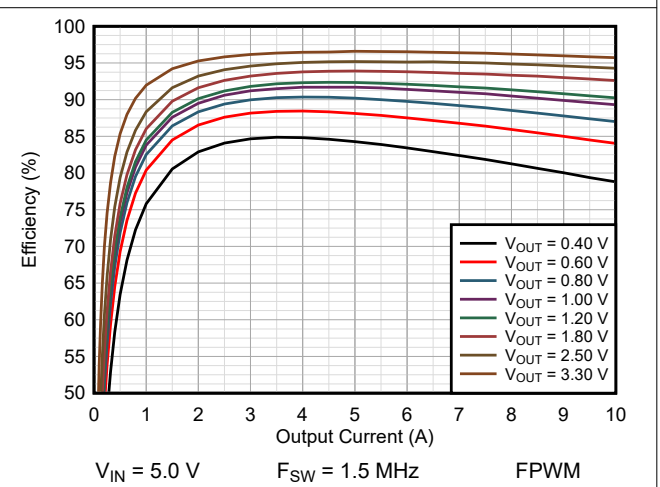
图 9-7. Efficiency TPSM8287A10BAH
