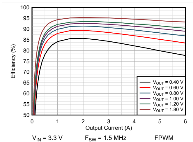
图 9-4. Efficiency TPSM8287A06BAS
