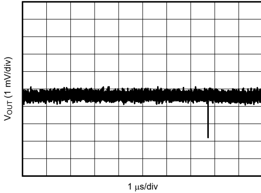
图 5-7. 第 2 个 L-C 滤波器之后的 V_{OUT} 纹波
