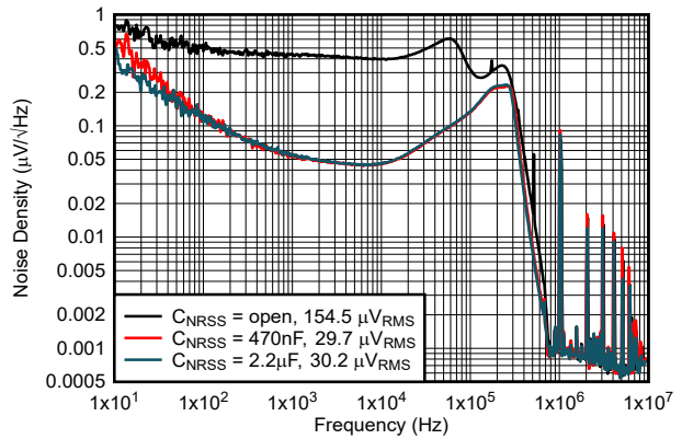
12V 至 1.2V 1 \mu H, 1MHz 铁氧体磁珠滤波器后 NR/SS = 开路, 470nF, 2.2 \mu F, BW = 100Hz 至 100kHz
