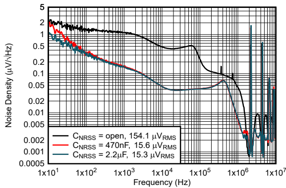
12V 至 3.3V 1 \mu H, 2.2MHz 仅第 1 个 L-C NR/SS = 开路, 470nF, 2.2 \mu F, BW = 100Hz 至 100kHz
