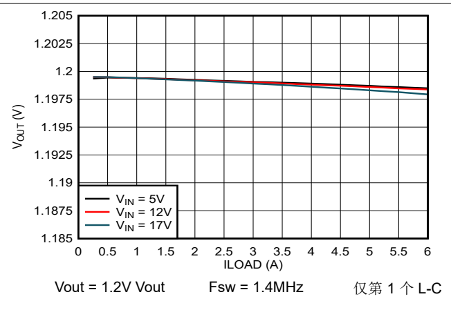
图 7-5. 输出电压与负载电流间的关系
