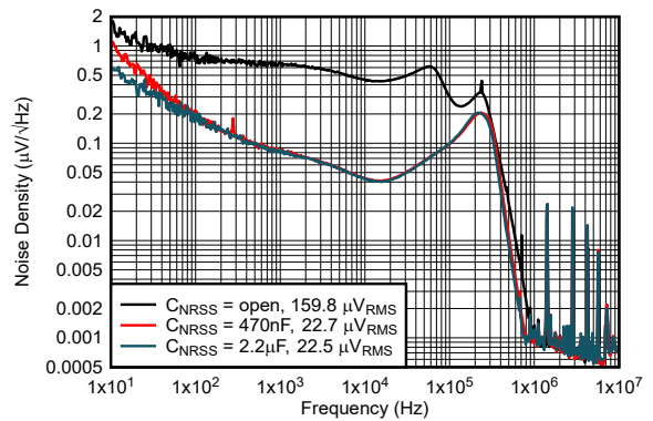
12V 至 1.8V 1 \mu H, 1.4MHz 铁氧体磁珠滤波器后 NR/SS = 开路, 470nF, 2.2 \mu F, BW = 100Hz 至 100kHz
