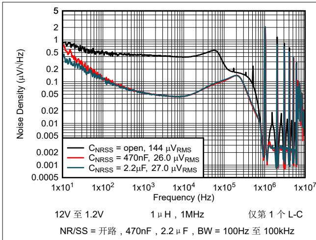
图 5-13. 输出噪声密度与频率间的关系
