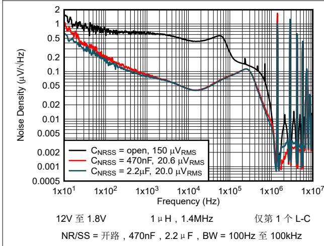
图 5-15. 输出噪声密度与频率间的关系
