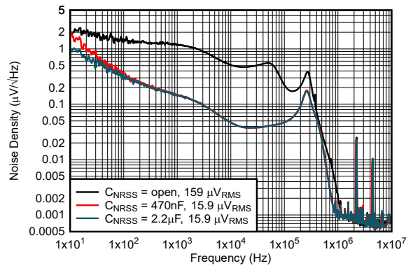
12V 至 3.3V 1 \mu H, 2.2MHz 铁氧体磁珠滤波器后 NR/SS = 开路, 470nF, 2.2 \mu F, BW = 100Hz 至 100kHz
