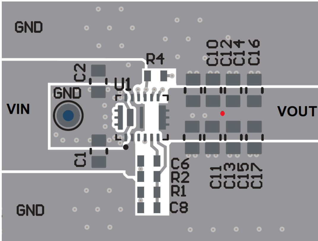
图 7-2. 单个 L-C 滤波器的建议布局
