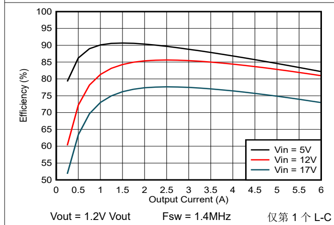
图 7-4. 效率与负载电流间的关系
