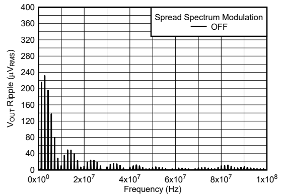
12V 至 1.8V, 2A 1 μH, 1.4MHz 仅第 1 个 L-C BW = 10kHz
