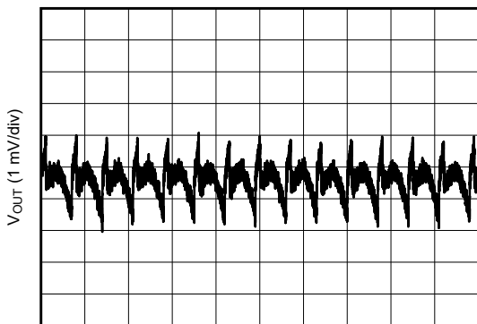
12V 至 1.8V, 2A 1 μH, 1.4MHz 仅第 1 个 L-C
