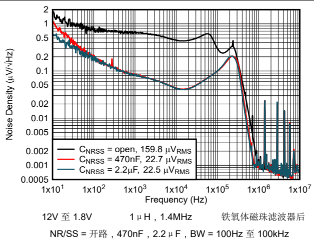
图 5-16. 输出噪声密度与频率间的关系
