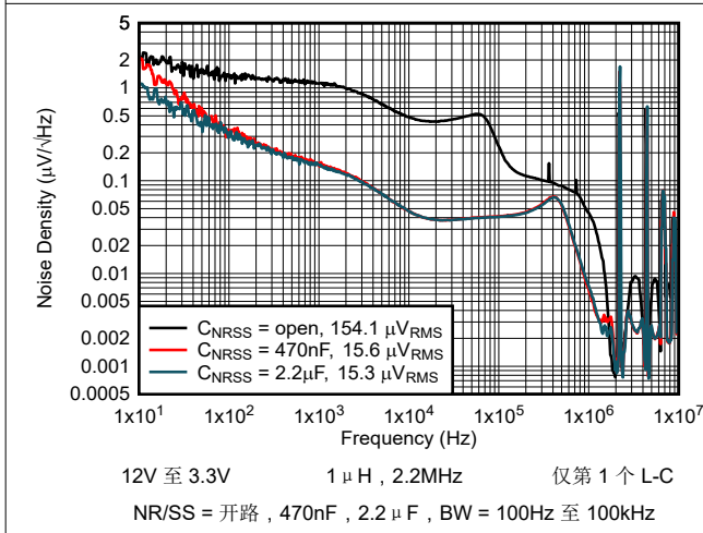
图 5-17. 输出噪声密度与频率间的关系
