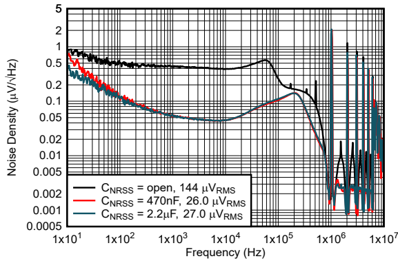
12V 至 1.2V 1 \mu H, 1MHz 仅第 1 个 L-C NR/SS = 开路, 470nF, 2.2 \mu F, BW = 100Hz 至 100kHz
