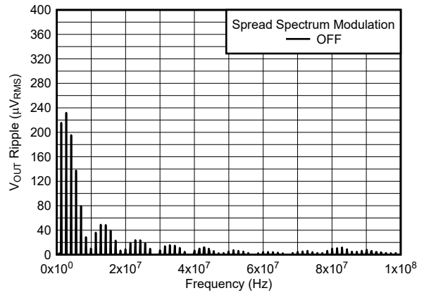
图 5-4. 第 2 个 L-C 滤波器之后的 V_{OUT} 纹波 FFT
