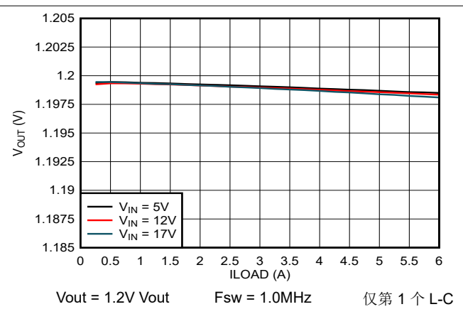
图 7-7. 输出电压与负载电流间的关系
