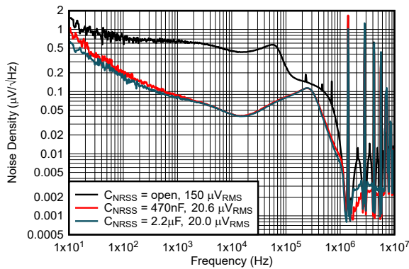
12V 至 1.8V 1 \mu H, 1.4MHz 仅第 1 个 L-C NR/SS = 开路, 470nF, 2.2 \mu F, BW = 100Hz 至 100kHz
