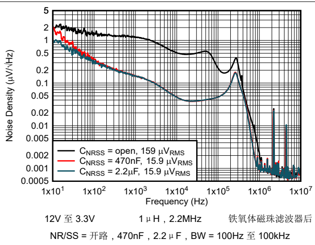
图 5-18. 输出噪声密度与频率间的关系
