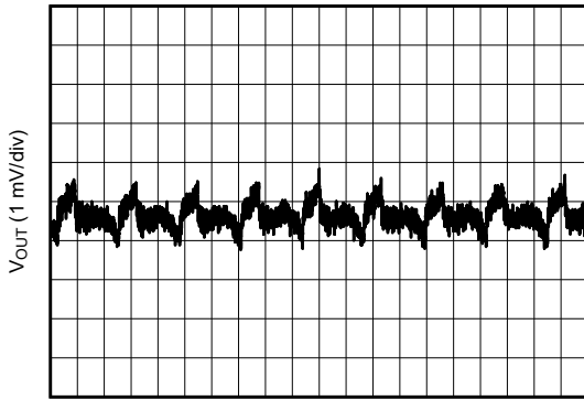
图 5-7. 第 2 个 L-C 滤波器之后的 V_{OUT} 纹波
