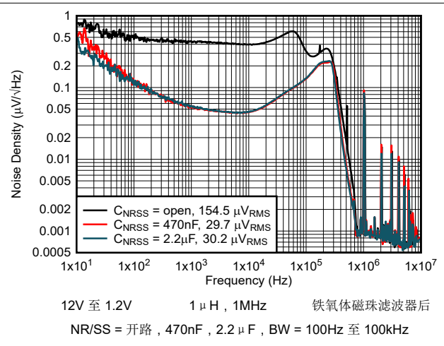
图 5-14. 输出噪声密度与频率间的关系
