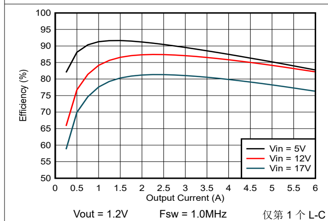
图 7-6. 效率与负载电流间的关系
