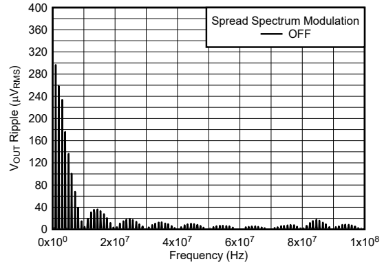
12V 至 1.2V, 2A 1 μH, 2MHz 仅第 1 个 L-C BW = 10kHz
