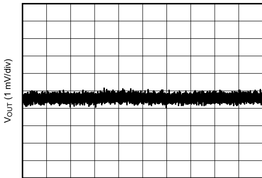
12V 至 1.2V, 2A 1 μH, 1MHz 第 1 和第 2 个 L-C
