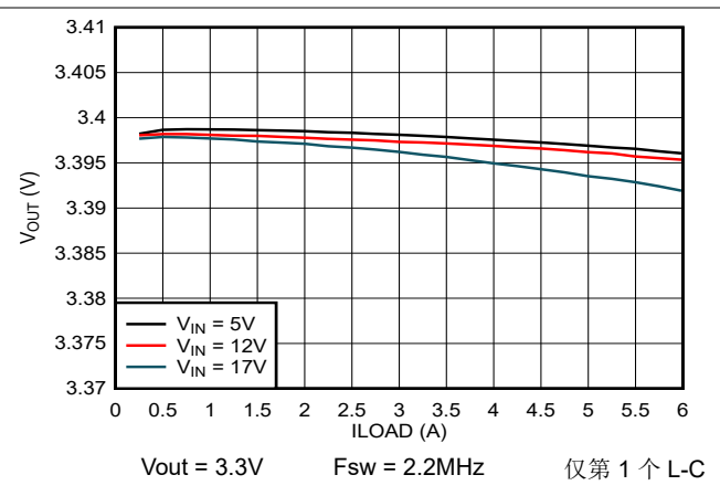
图 7-3. 输出电压与负载电流间的关系
