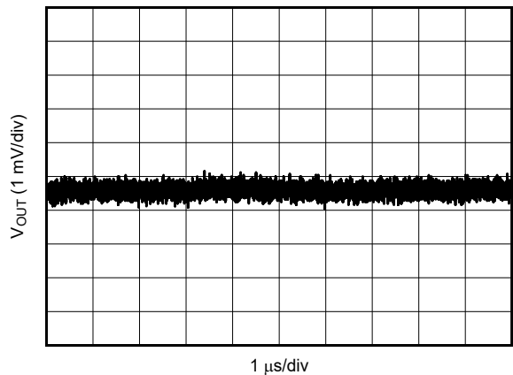
图 5-3. 第 2 个 L-C 滤波器之后的 V_{OUT} 纹波
