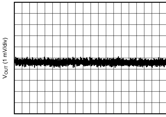
图 5-9. 第 1 个 L-C 滤波器之后的 V_{OUT} 纹波
