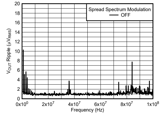
12V 至 1.2V, 2A 1 μH, 1MHz 第 1 和第 2 个 L-C BW = 10kHz
