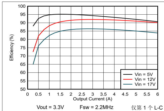
图 7-2. 效率与负载电流间的关系
