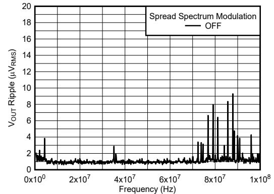
图 5-10. 第 1 个 L-C 滤波器之后的 V_{OUT} 纹波 FFT
