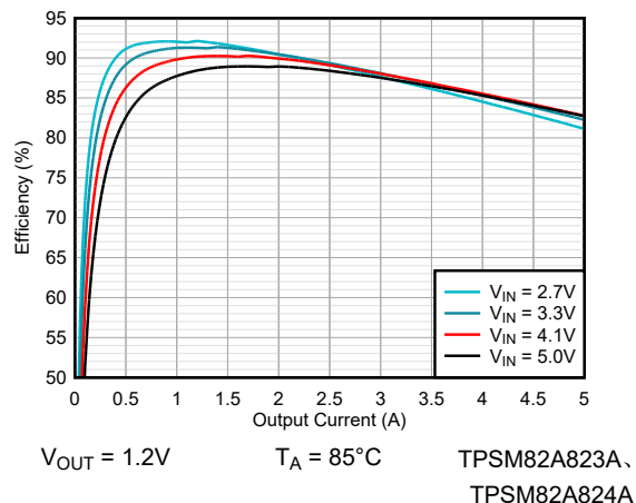
图 8-33. 效率
