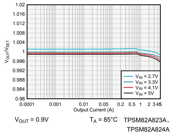
图 8-47. VOUT 精度
