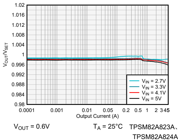
图 8-48. VOUT 精度
