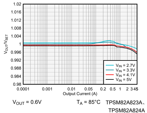
图 8-49. VOUT 精度
