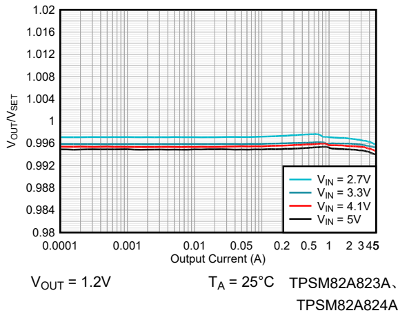
图 8-44. VOUT 精度
