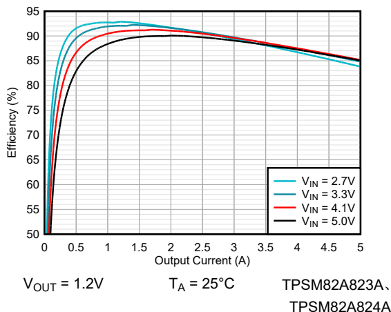
图 8-32. 效率
