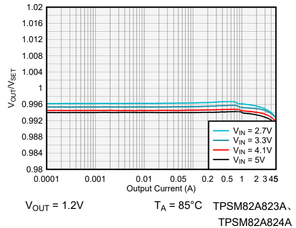
图 8-45. VOUT 精度
