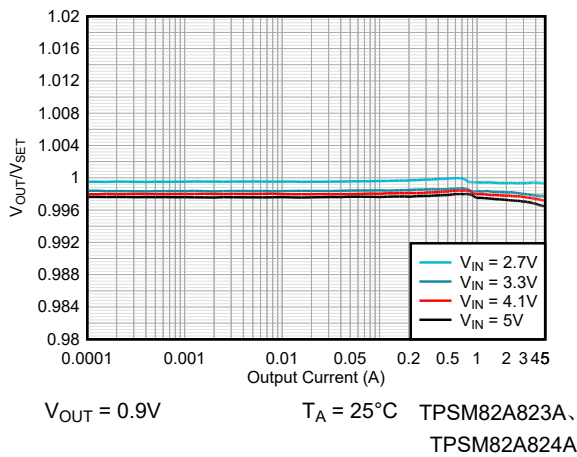
图 8-46. VOUT 精度
