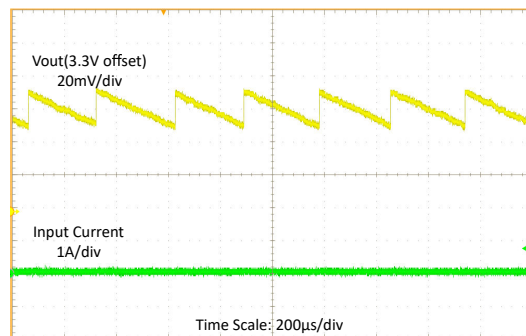
图 8-9. 负载为 1mA 时的开关波形
