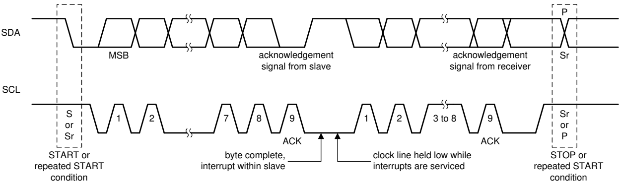
图 7-7. 总线协议
