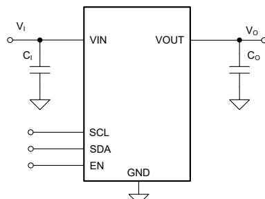
典型应用
