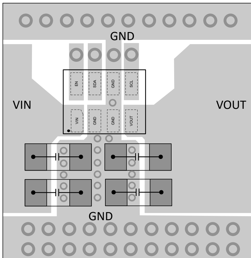
图 9-1. 布局示例
