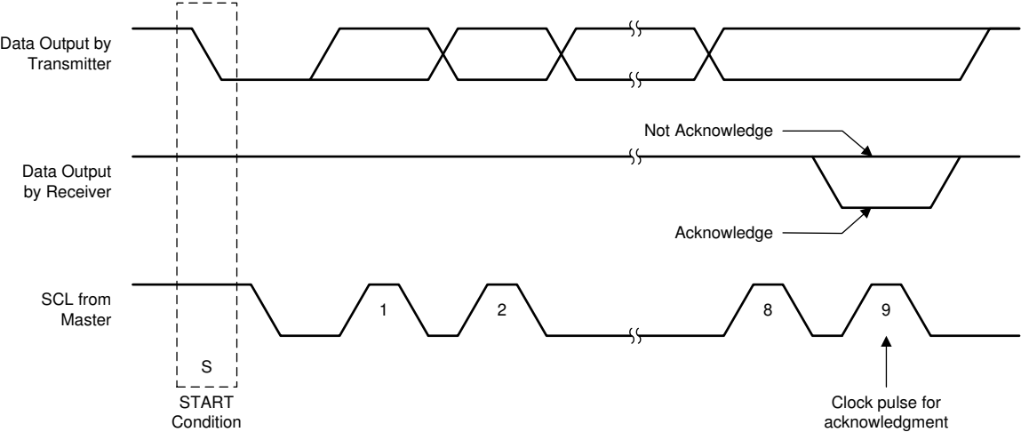
图 7-6. I 2 C 总线上的确认
