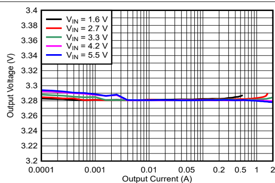
图 8-3. 负载调节 (FPWM)
