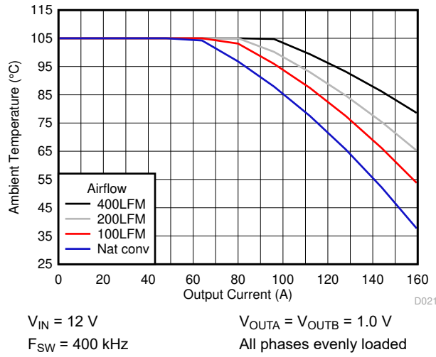
图 6-7. Thermal Safe Operating Area
