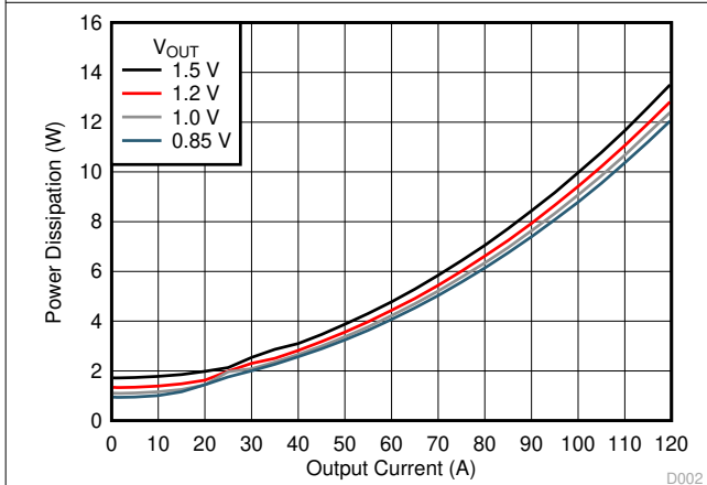
图 6-3. VOUTA Power Dissipation
