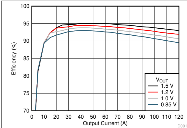
图 6-1. VOUTA Efficiency
