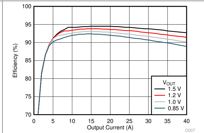
图 6-2. VOUTB Efficiency
