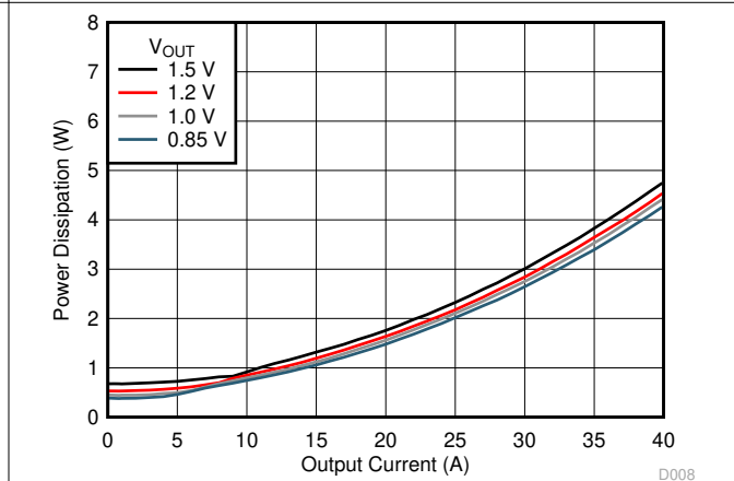
图 6-4. VOUTB Power Dissipation
