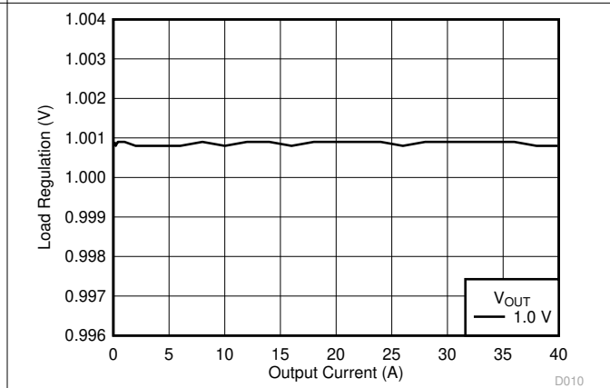
图 6-6. VOUTB Load Regulation
