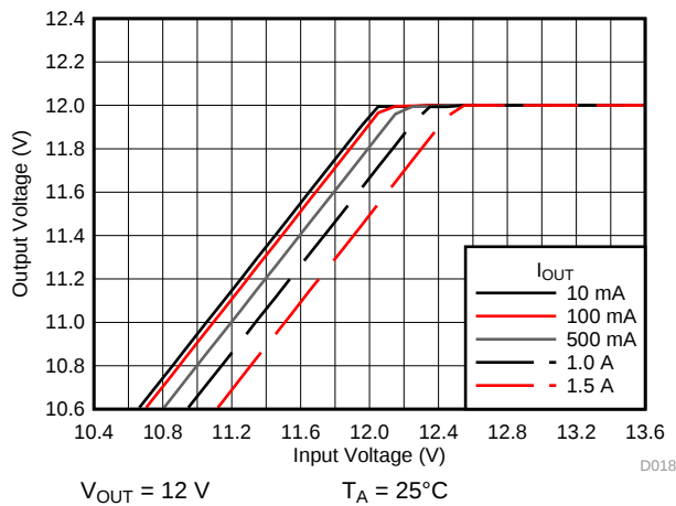
图 18. Drop-Out Voltage
