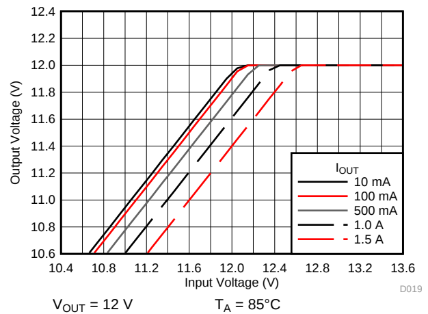
图 19. Drop-Out Voltage
