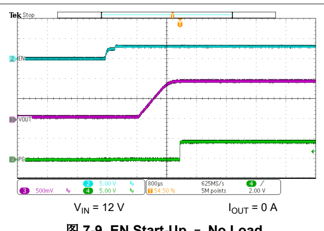
图 7-9. EN Start-Up - No Load
