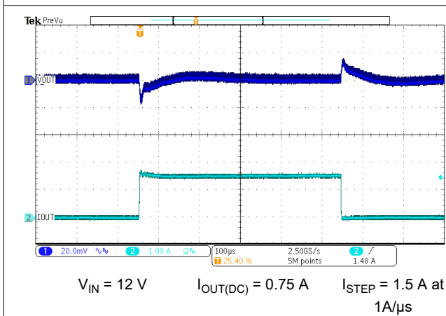
图 7-8. Load Transient
