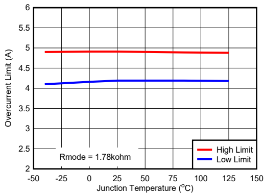
图 5-3. Overcurrent Limit : R = 1.78kOhm
