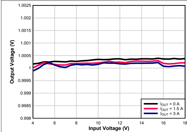
图 7-6. Line Regulation
