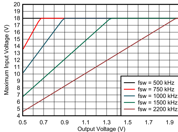
图 7-2. Maximum Input Voltage vs Output Voltage
