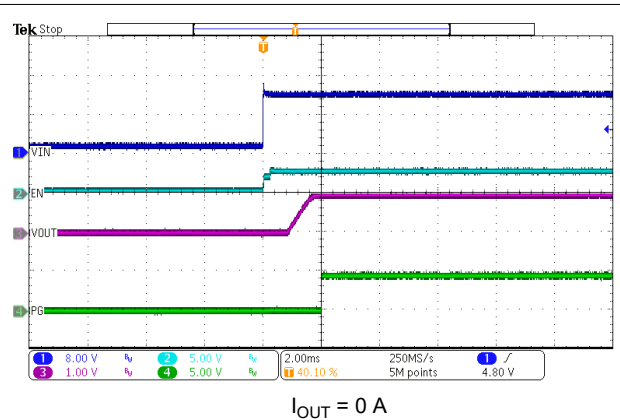
图 7-13. VIN Start-Up
