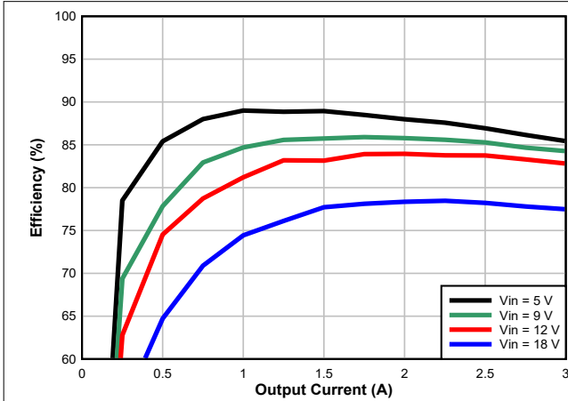
图 7-4. Efficiency
