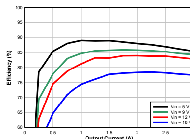
效率
