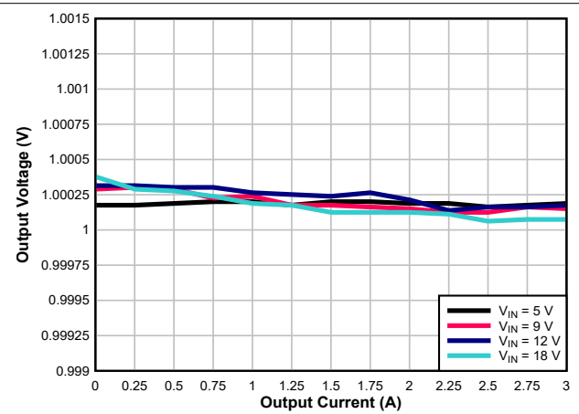
图 7-5. Load Regulation
