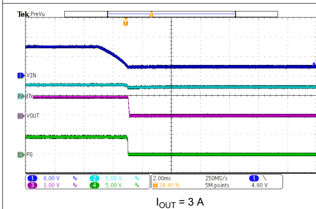
图 7-14. VIN Shutdown
