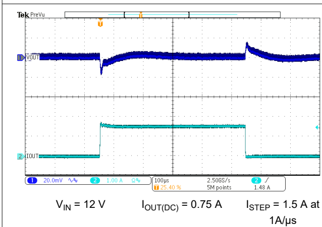
图 7-8. Load Transient
