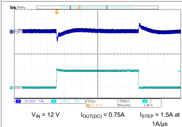
图 7-8. Load Transient
