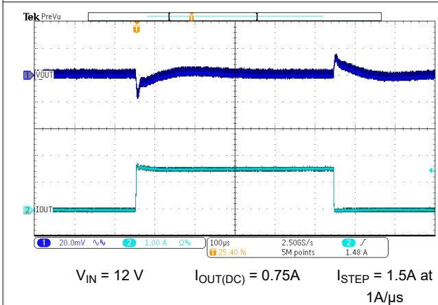
图 7-8. Load Transient
