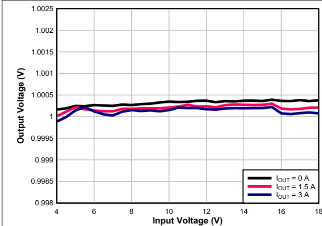
图 7-6. Line Regulation
