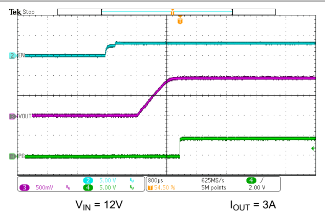
图 7-11. EN Start-Up – With Load
