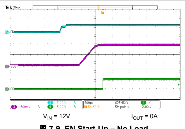
图 7-9. EN Start-Up – No Load
