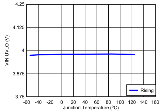
图 5-8. Vin UVLO
