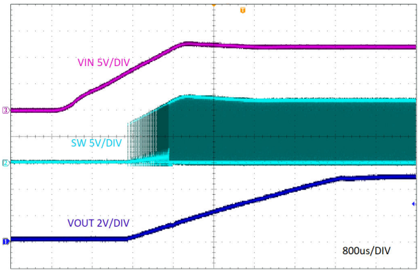
图 7-3. 相对于 V_{IN} 、 I_{OUT} = 3A 的启动
