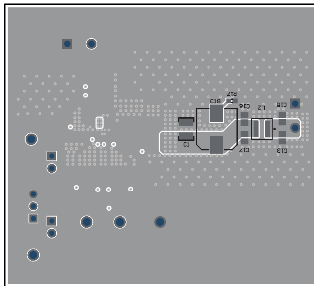
图 7-10. TPSM843521 底层布局示例
