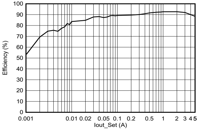
图 7-2. 效率 (PFM)
