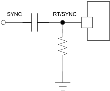
图 6-3. SYNC 模式配置
