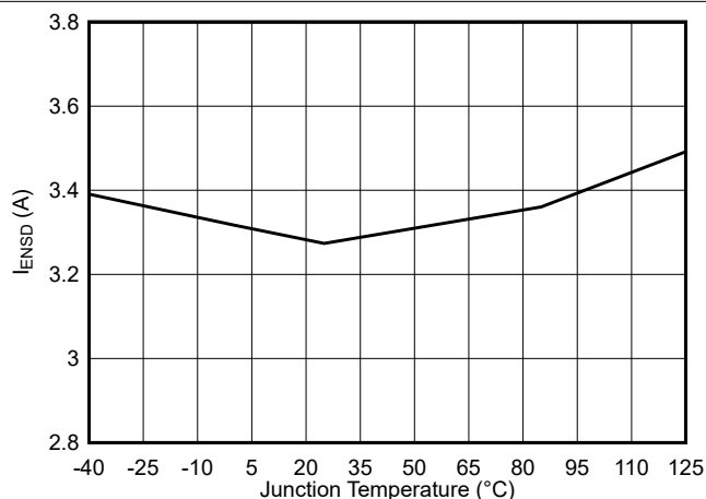
图 5-2. TPSM843521 关断电流与结温间的关系
