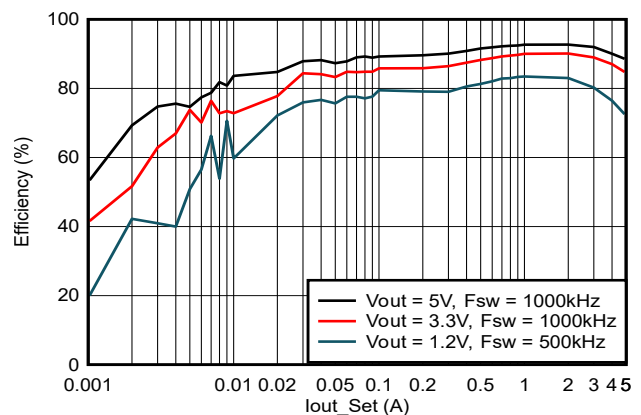
TPSM843521 效率, PFM
