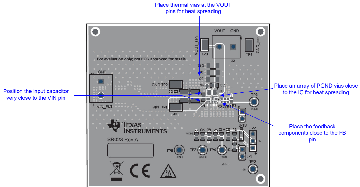
图 7-9. TPSM843521 顶层布局示例
