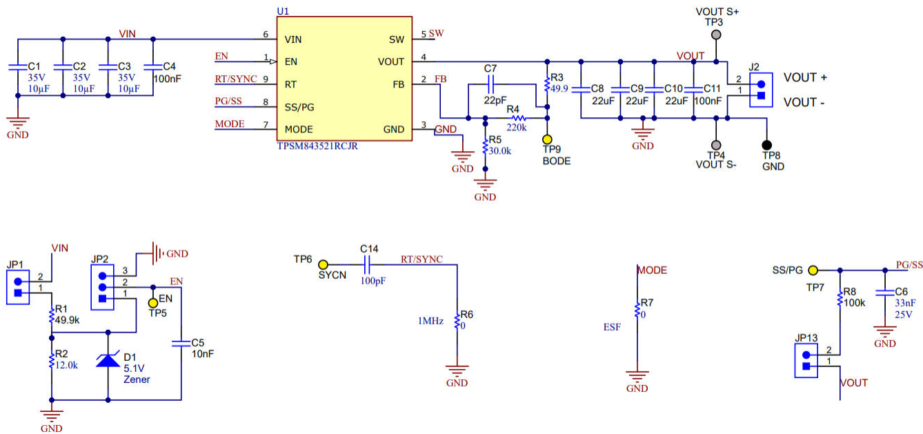
图 7-1. TPSM843521 5V 输出、5A 参考设计
